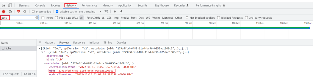
图 8-7 获取 job_id
