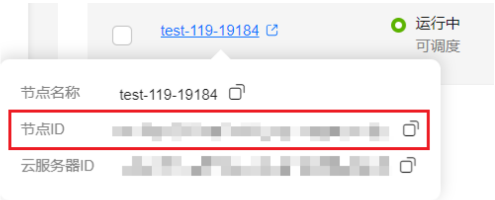
图 8-4 获取 node_id
