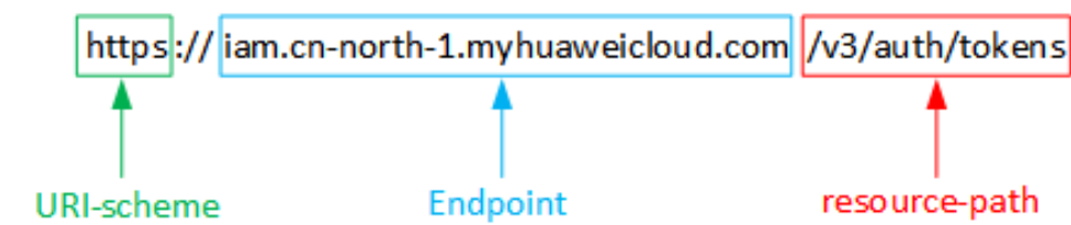
图 3-1 URI 示意图
