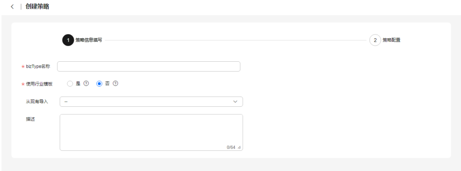
图 6-5 创建策略
