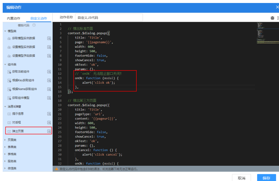
图 4-33 自定义 JS 代码
