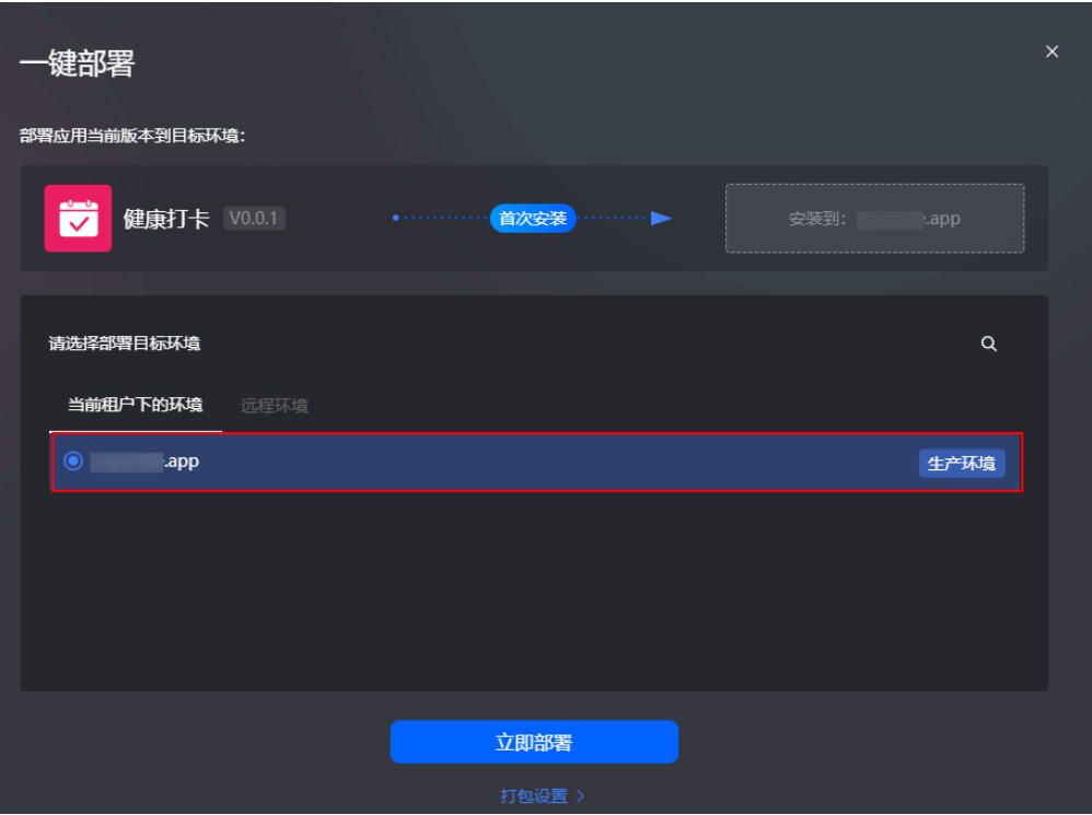
图 4-54 一键部署
