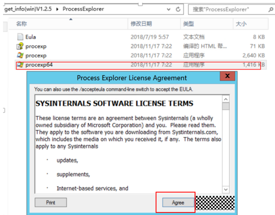
图 5-3 processExplorer
