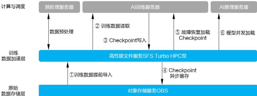
图 2-1 基于 OBS+SFS Turbo 的华为云 AI 云存储解决方案
