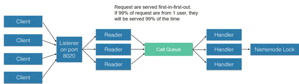
图 6-12 基于 FIFO 调用队列的 NameNode 请求处理
