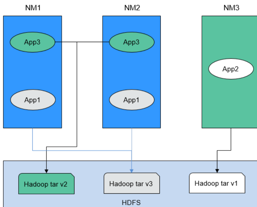
图 15-1 具有多个版本 NodeManagers 及 Applications 的集群
