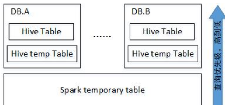
图 20-11 Spark 表管理层次
