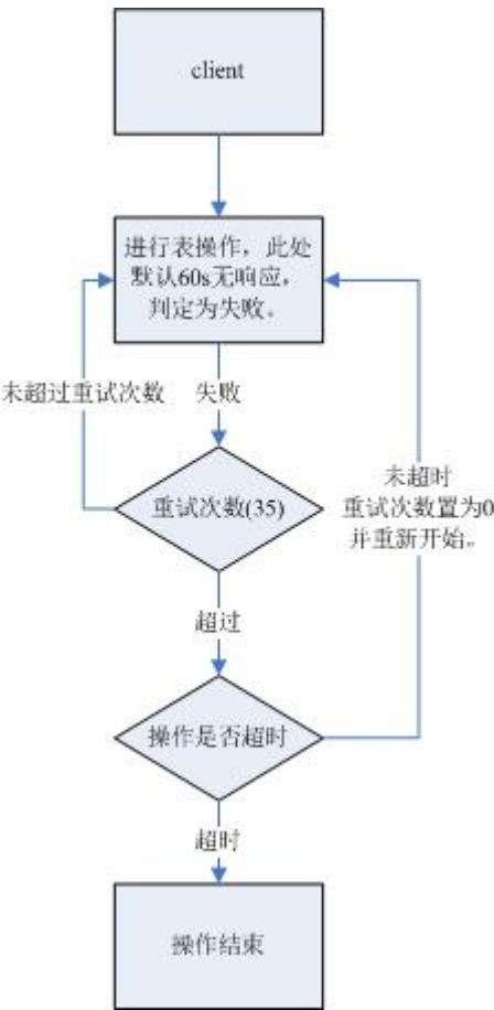
图 5-3 HBase 客户端操作重试超时流程
