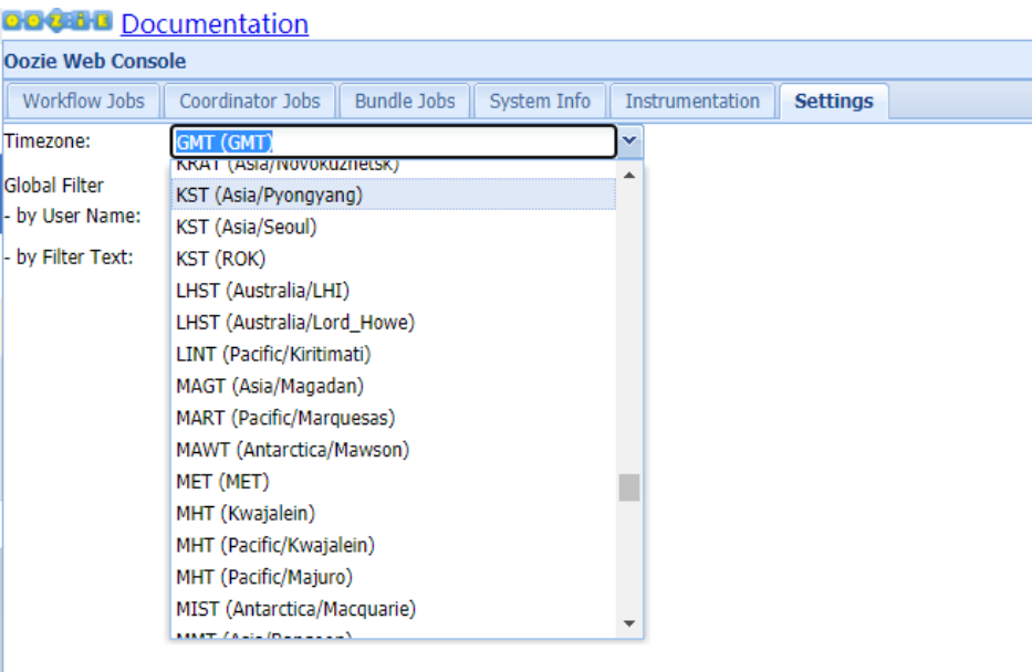
图 10-12 时区参考
