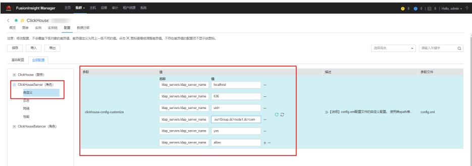
图 1-2 OpenLDAP 配置
