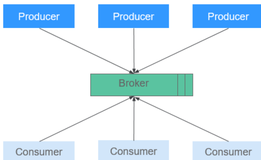
图 12-1 Kafka 结构
