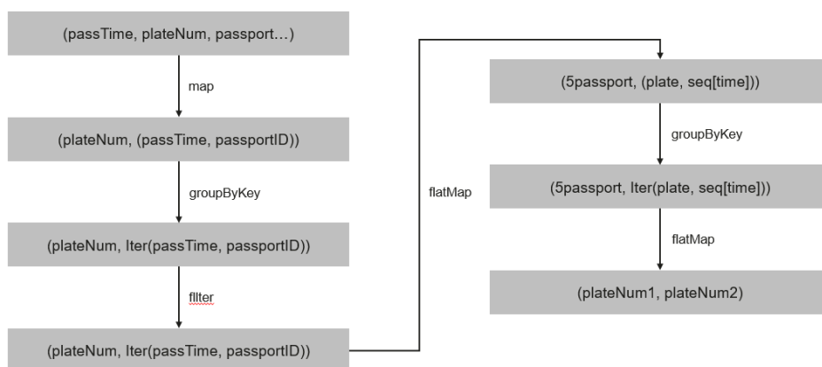
图 20-6 实现 2 逻辑
