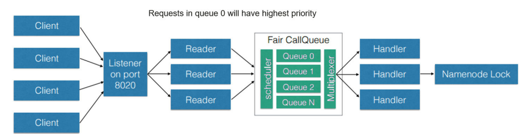
图 6-13 基于 FAIRCallQueue 的 NameNode 请求处理
