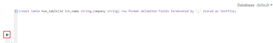
图 10-1 执行语句
