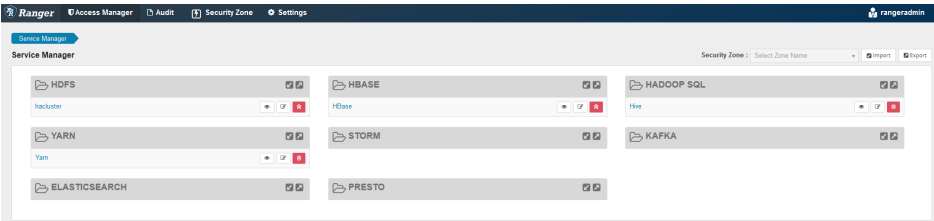
图 18-1 Ranger WebUI
