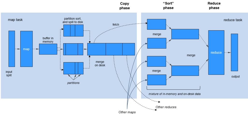
图 15-2 Shuffle 过程
