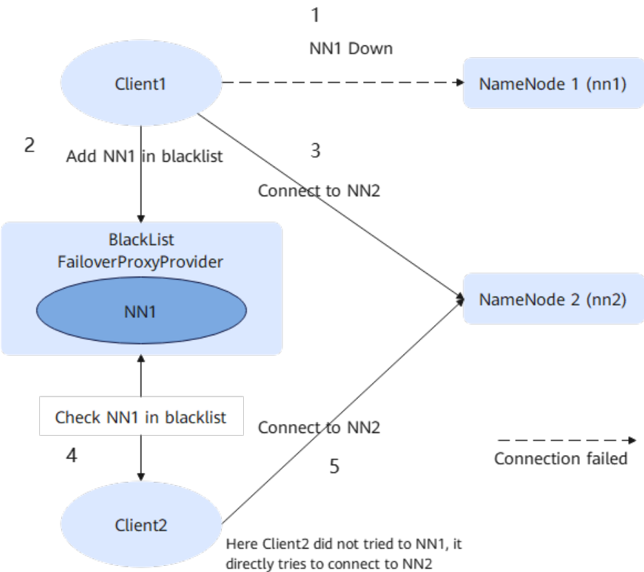
图 6-11 NameNode blacklisting 状态图
