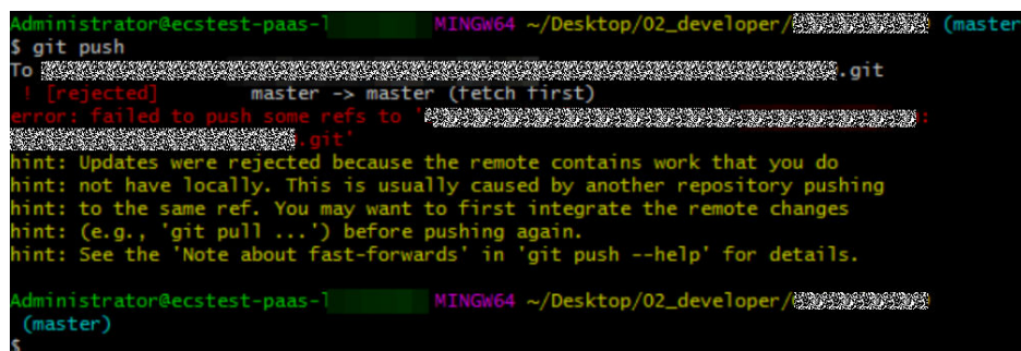
图 5-1 push 代码时报错信息图
