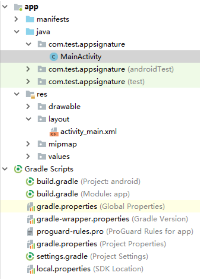
图 2-20 工程目录结构
