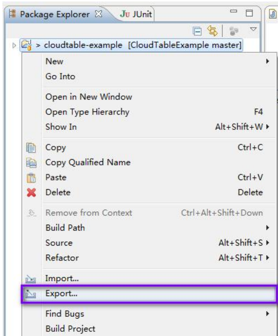
图 1-9 导出 Jar 包
