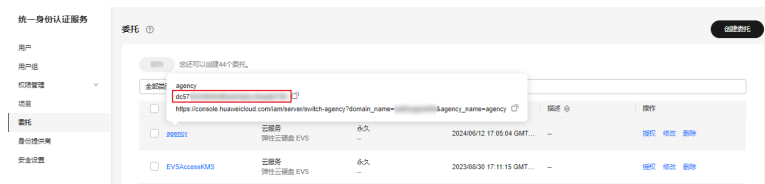
图 6-1 agency_id
