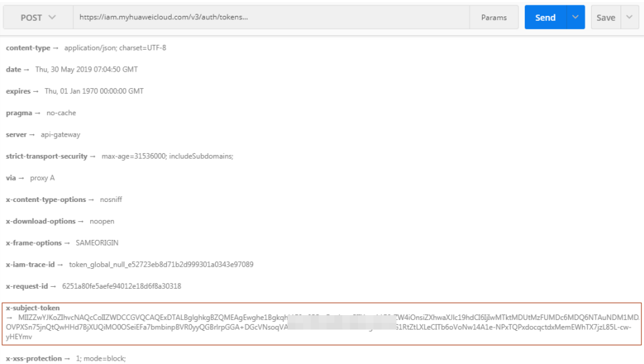
Figura 6-1 Obtención de un token de usuario
