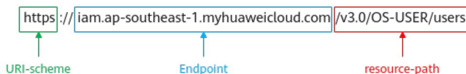
图 3-1 URI 示意图
