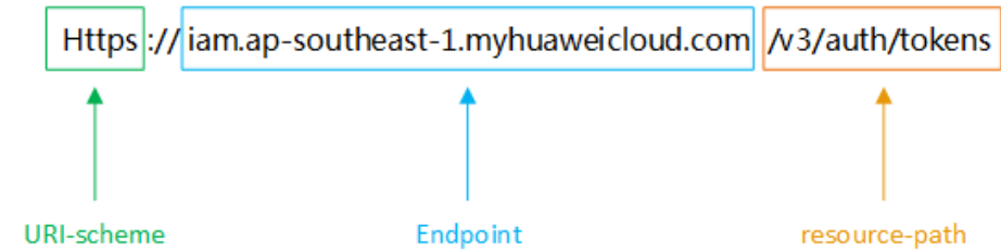
图 3-2 URI 示意图
