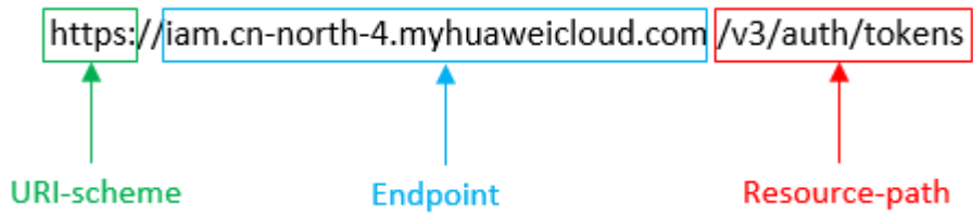
图 3-1 URI 示意图
