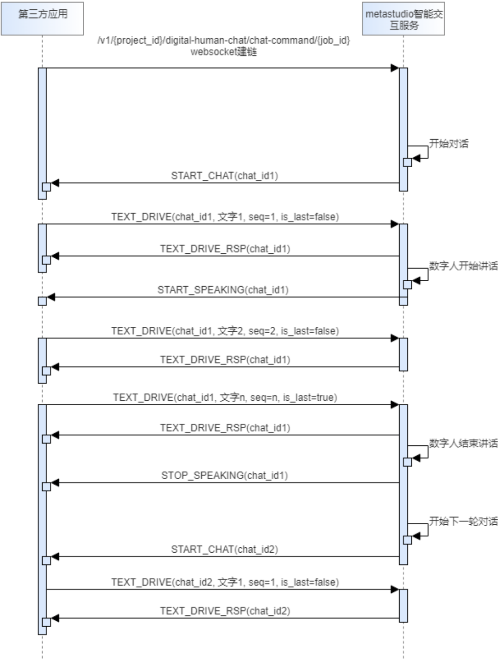
图 7-2 智能交互流式驱动流程图
