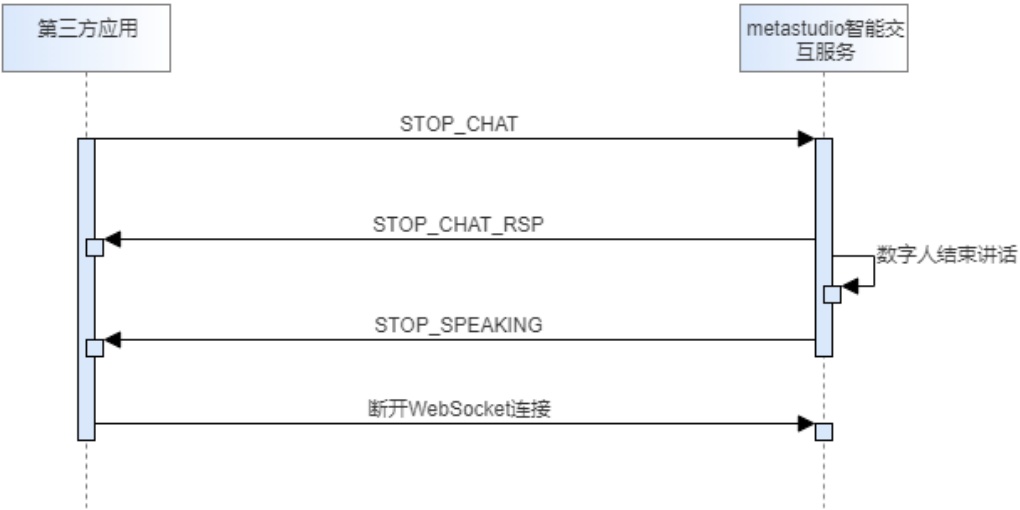
图 7-4 智能交互驱动停止对话流程图
