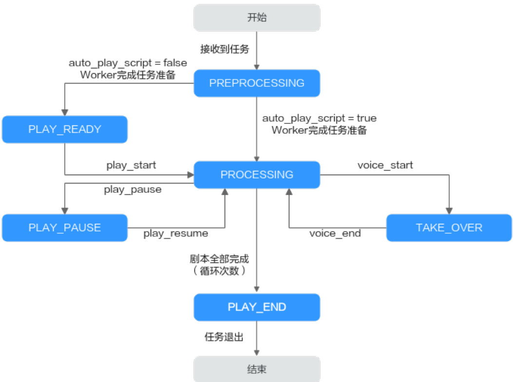
图 15-4 直播状态变化流程图
