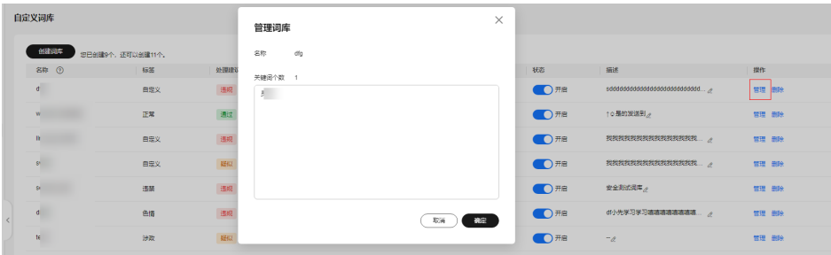
图 6-3 增加关键词
