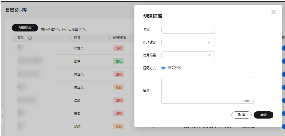
图 6-2 创建词库
