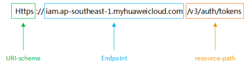
图 3-1 URI 示意图
