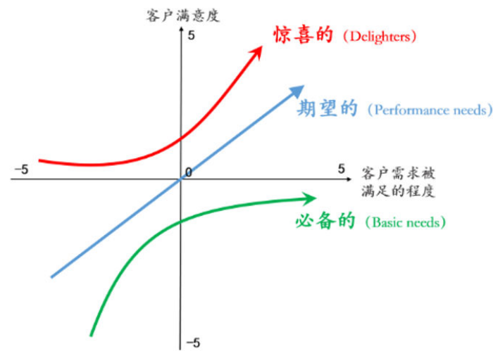
图 2-12 优先级模型
