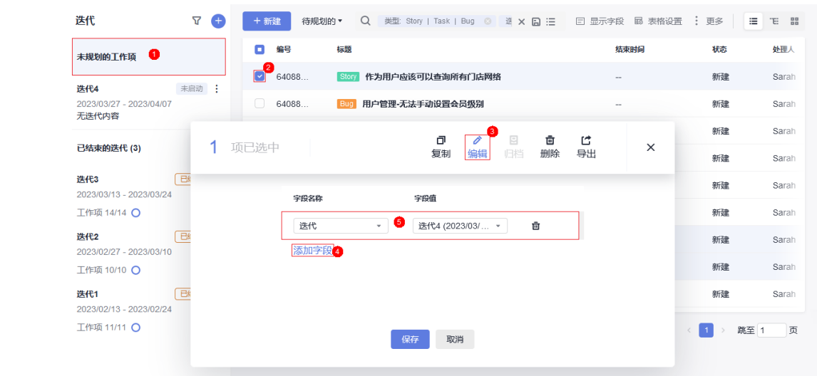
图 9-5 规划迭代
