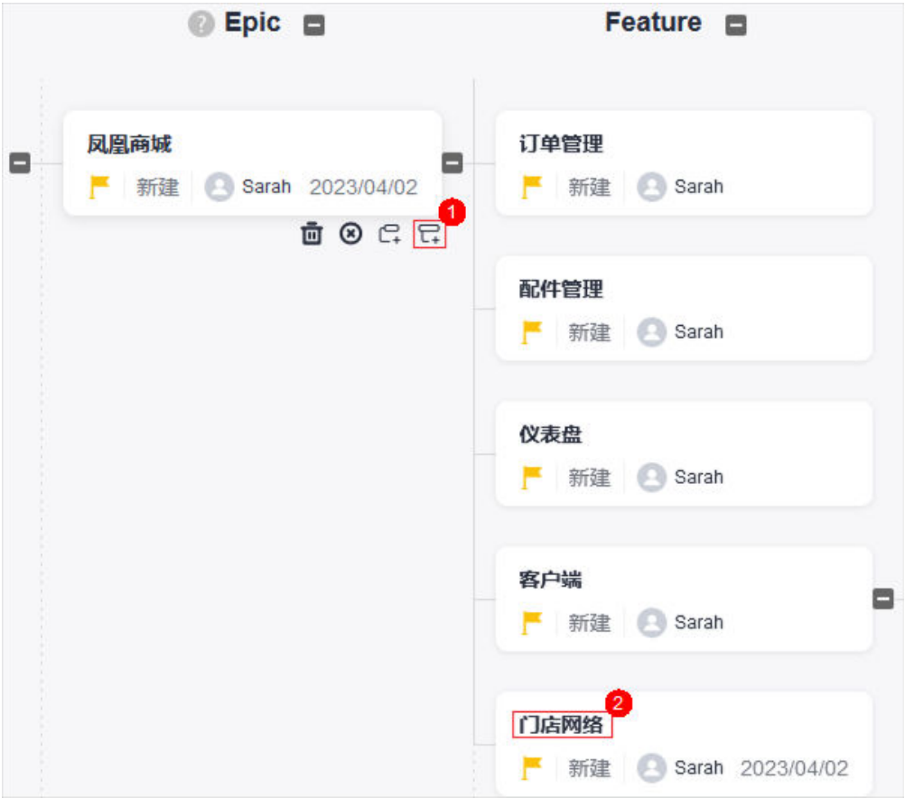
图 9-3 新建 Feature
