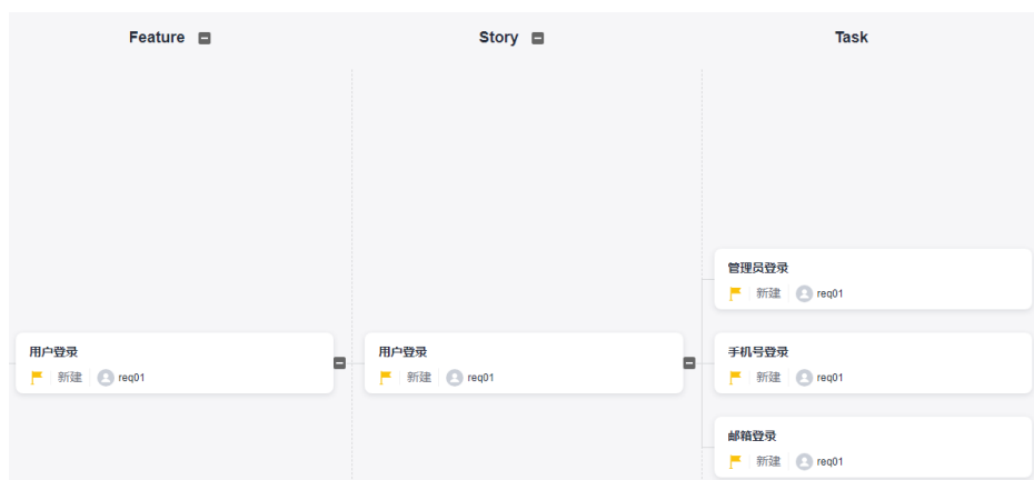
图 2-8 需求结构
