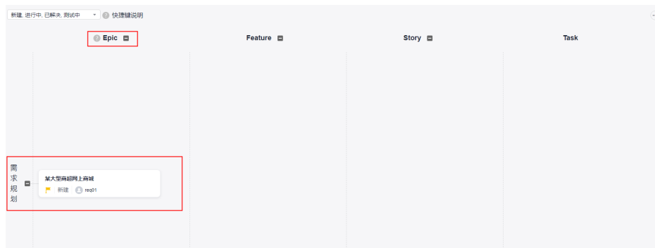
图 2-3 新建 Epic
