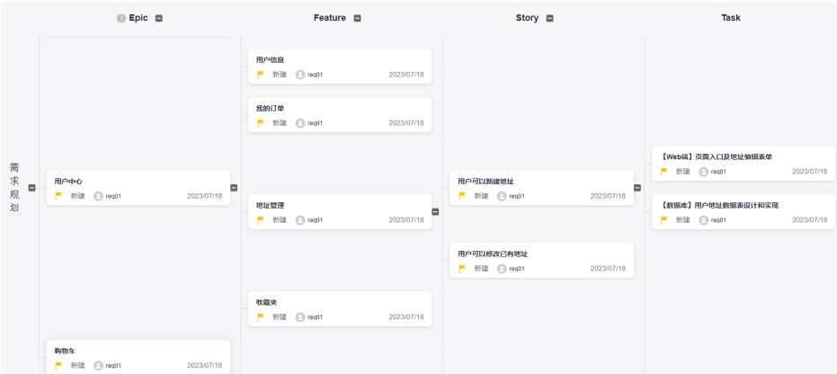
图 2-9 需求规划
