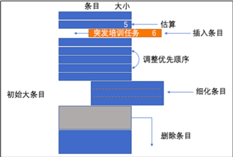
图 2-19 Backlog 结构
