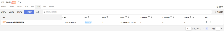
图 7-6 评审单列表
