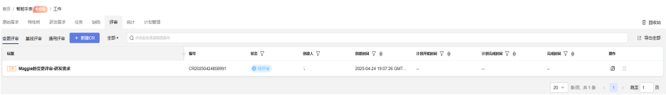
图 7-20 评审单列表
