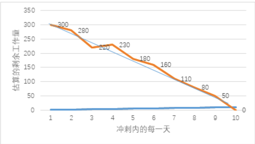
图 2-37 燃尽图
