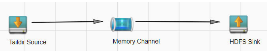
图 4-18 Flume 配置工具示例
