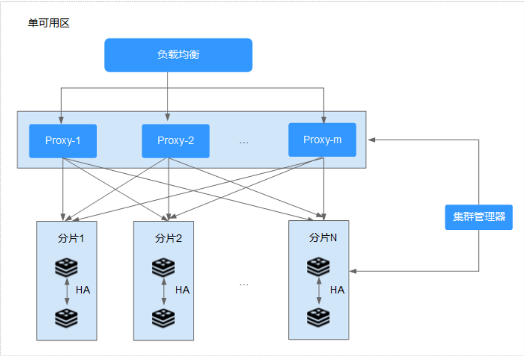
图 1-11 单可用区内集群版实例高可用
