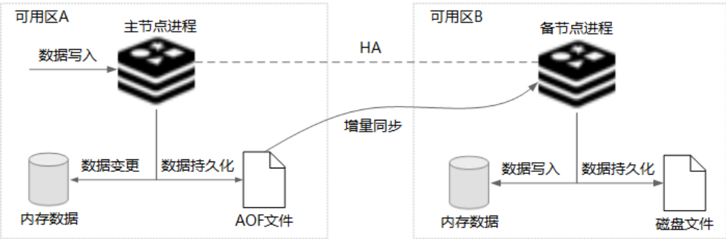
图 1-12 实例跨可用区示意图
