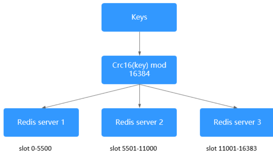
图 1-5 Redis Cluster 预分片示意图
