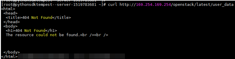
图 4-68 404 Not Found
