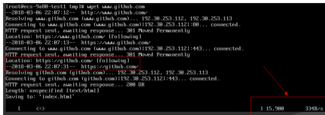
图 15-4 wget 下载包
