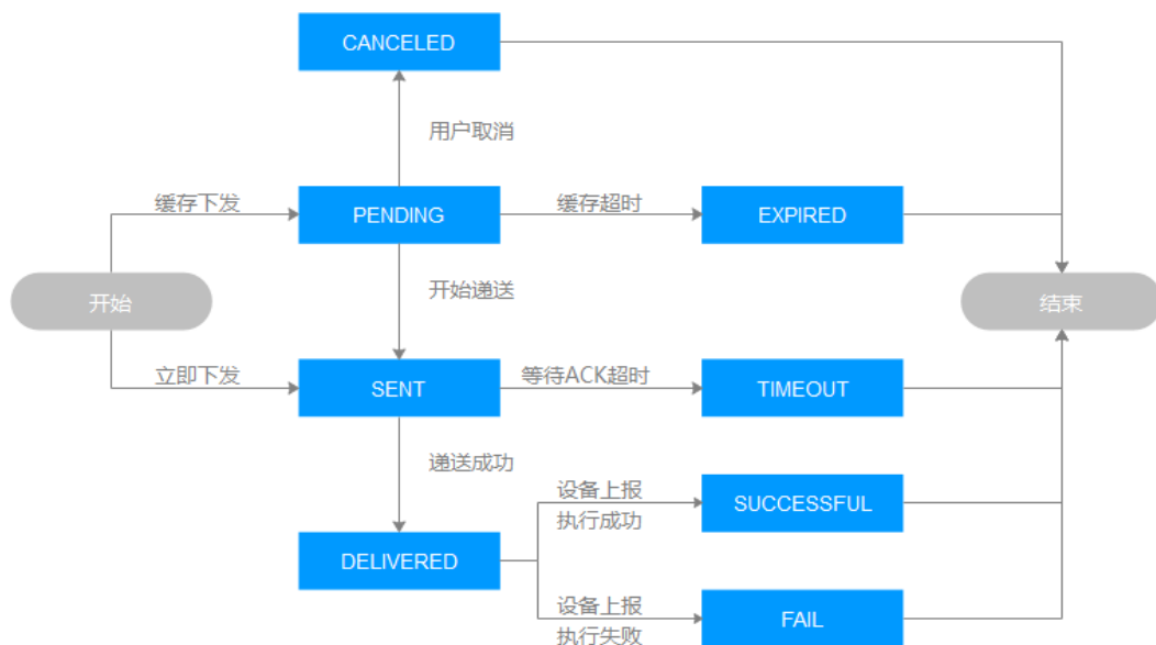
图 8-6 命令状态转换图
