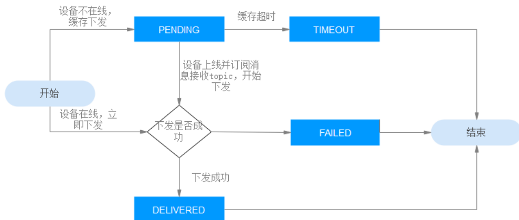
图 8-7 消息状态转换图
