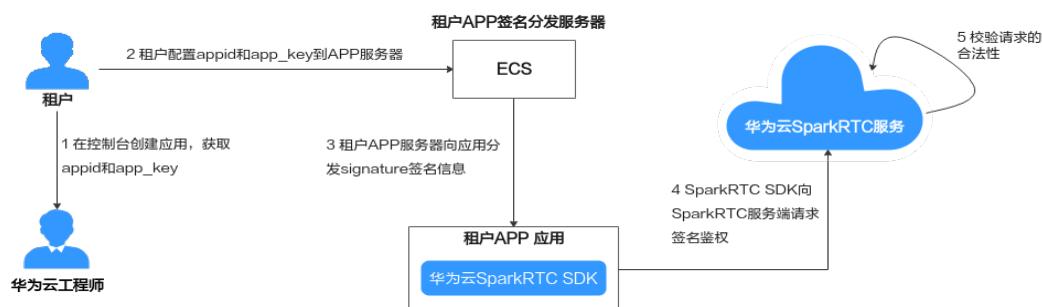
图 3-1 鉴权原理
