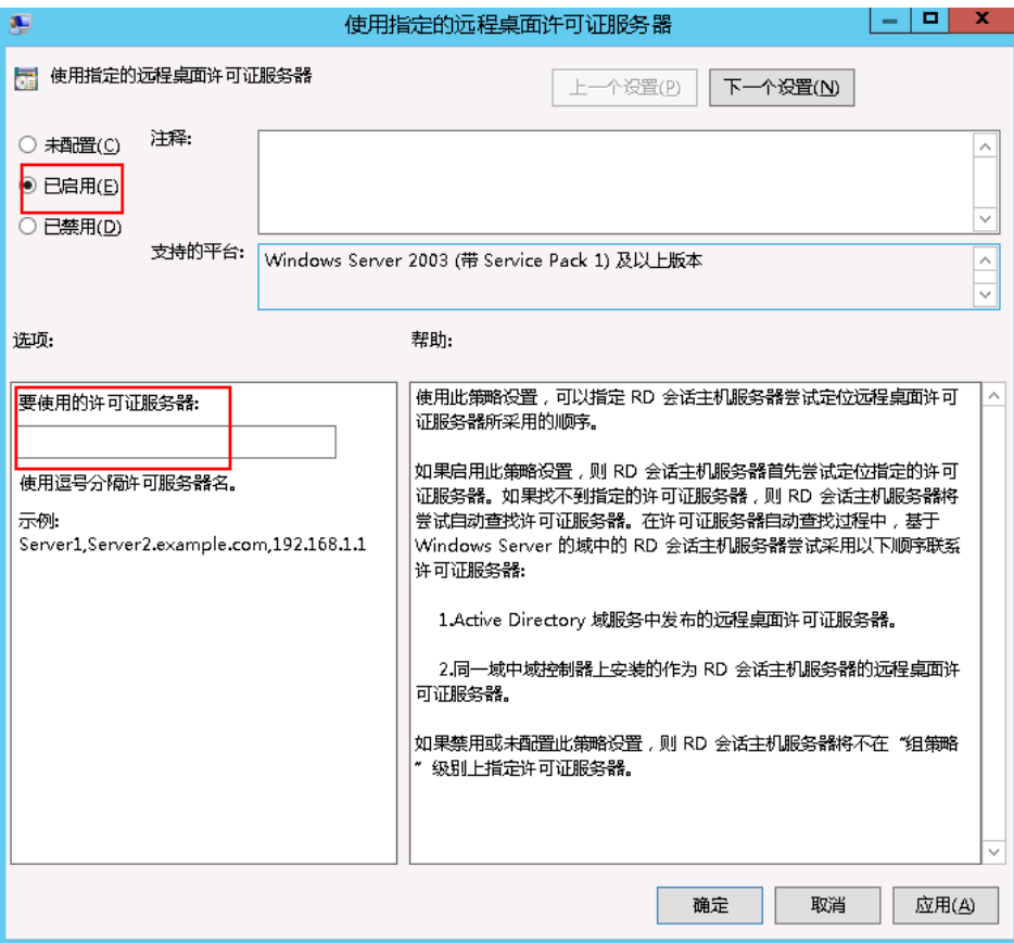
图 10-43 使用指定的远程桌面许可证服务器
