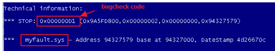
图 13-1 bugcheck code 以及可能的导致蓝屏的模块
