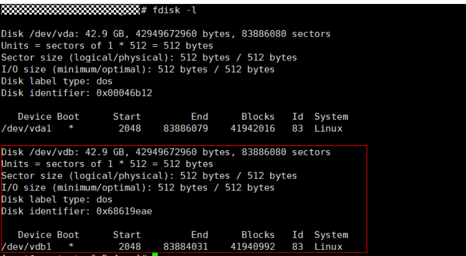
图 3-29 查看新增磁盘设备
