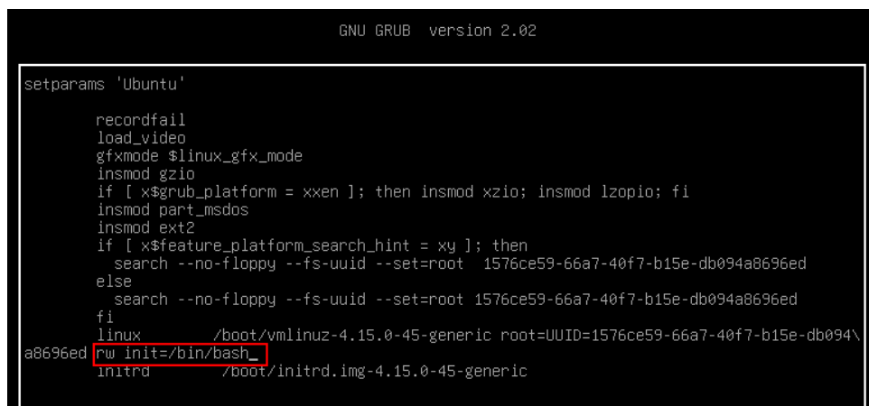
图 11-15 修改 ro 参数
