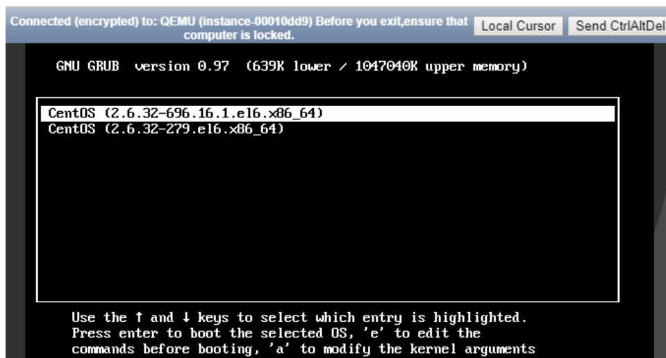
图 11-10 按字母键 e 编辑
