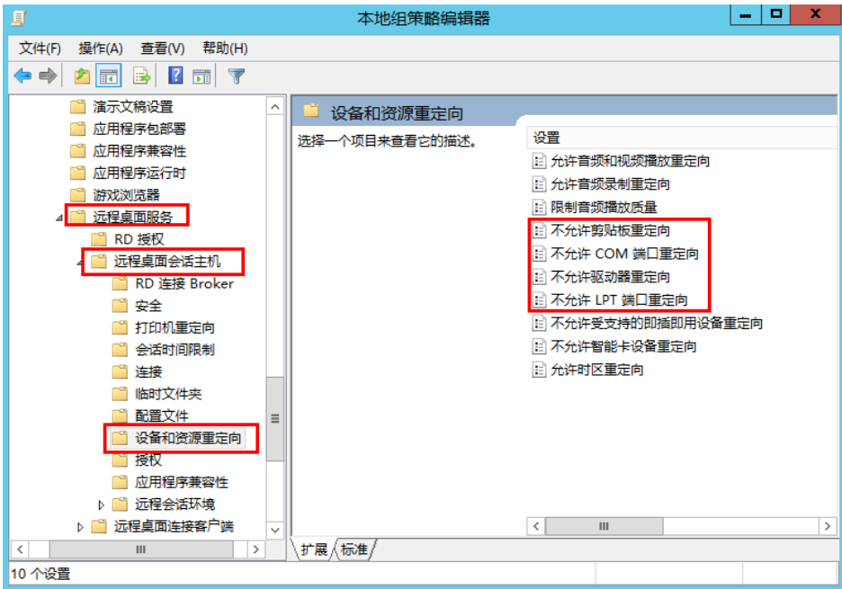
图 2-11 设备和资源重定向
