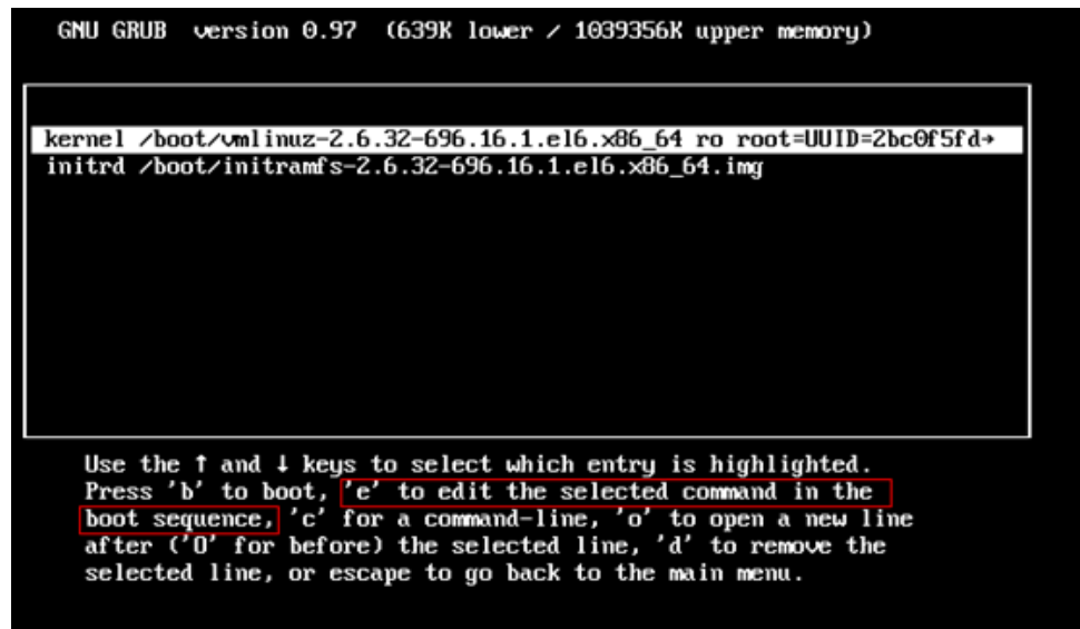
图 11-11 移动至 kernel 行
