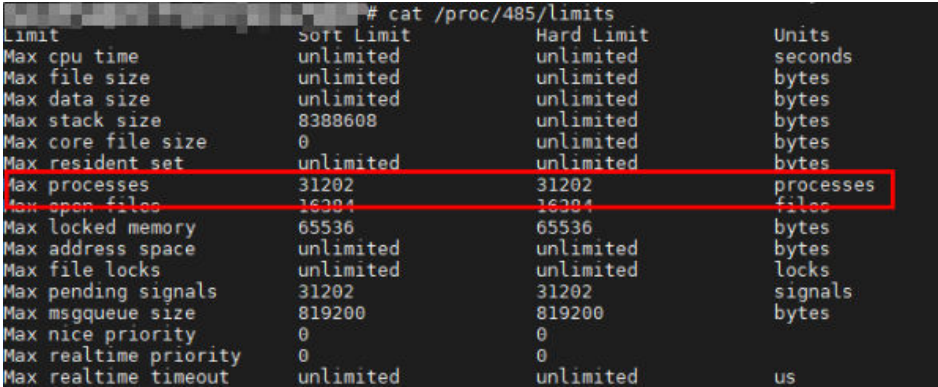
图 3-22 确定进程 limits 配置
