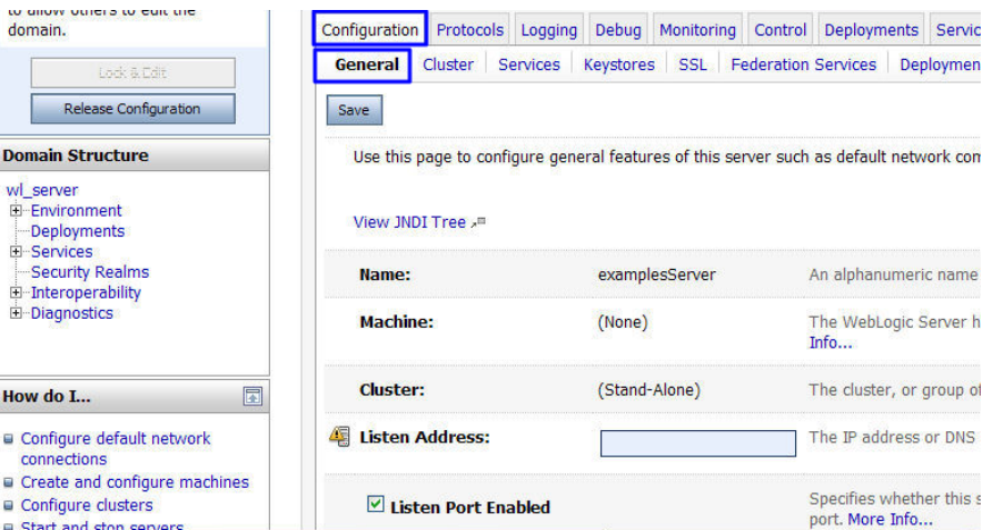
图 4-15 端口
