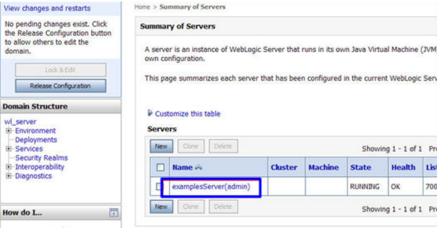
图 4-14 目标服务器
