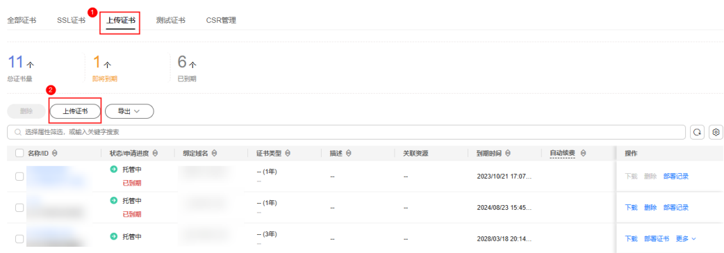
图 5-10 上传证书
