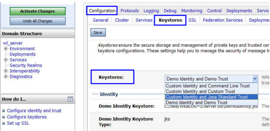
图 4-16 认证方式
