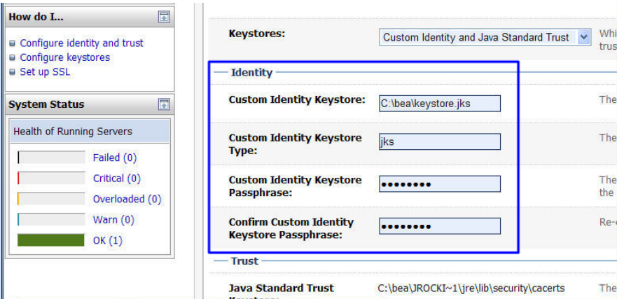
图 4-17 密钥
