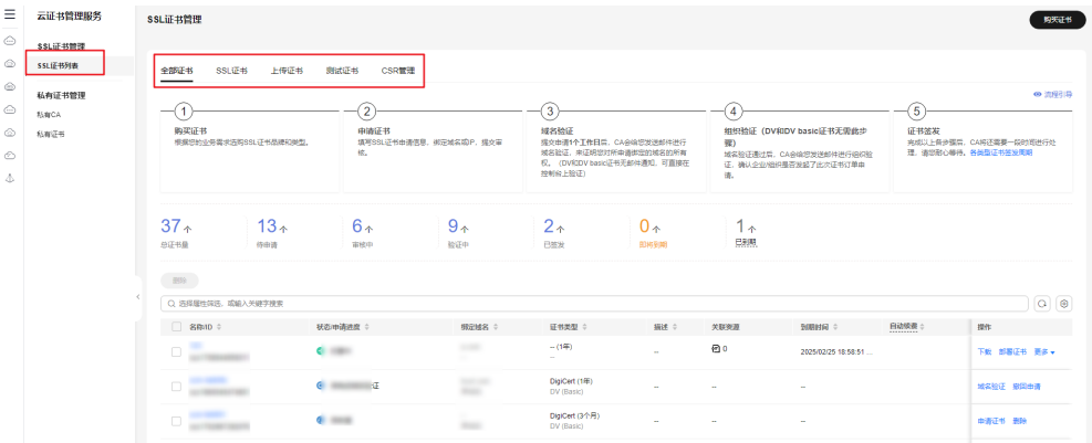
图 5-17 证书列表
