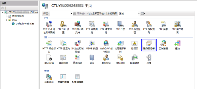
图 4-7 服务器证书
