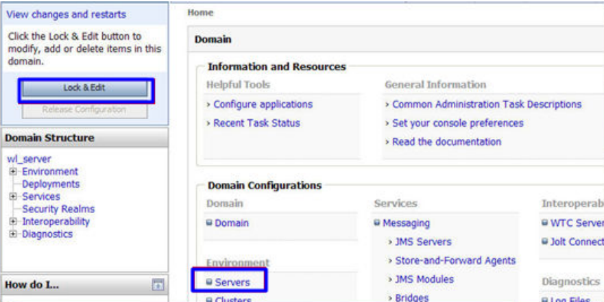
图 4-13 服务器
