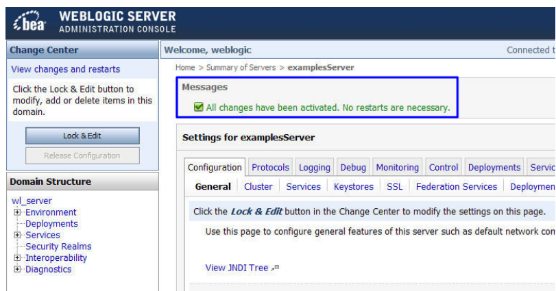
图 4-21 提示信息
