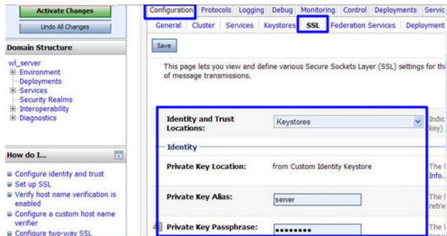
图 4-19 私钥
