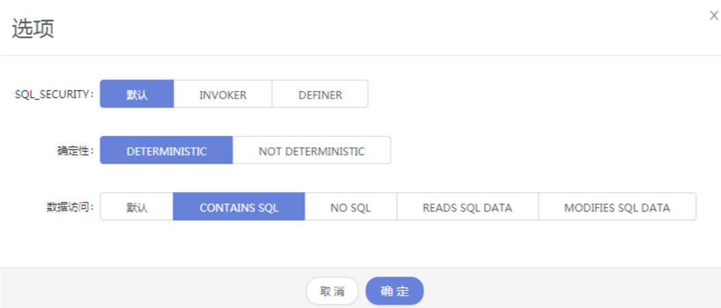
图 8-62 修改函数信息
