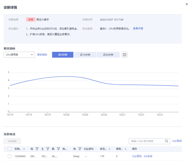
图 6-169 查看诊断详情
