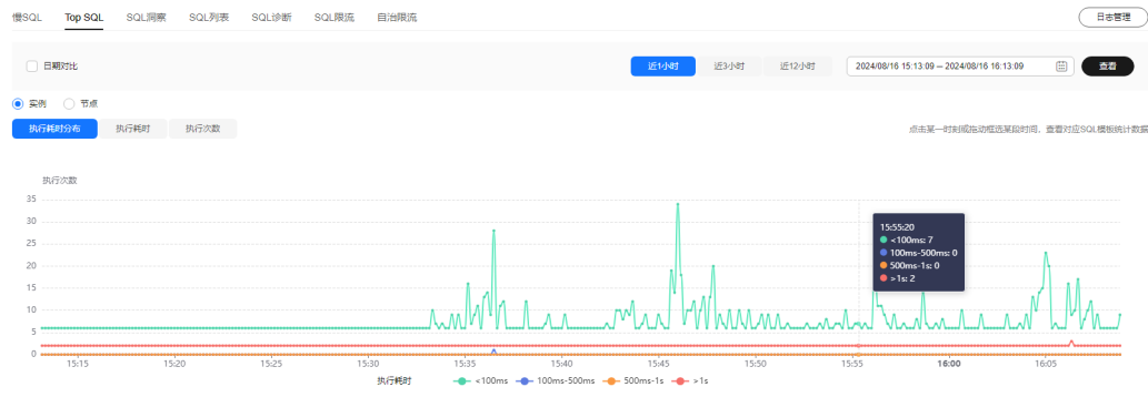
图 12-22 查看特定时间点的 TOP SQL 列表
