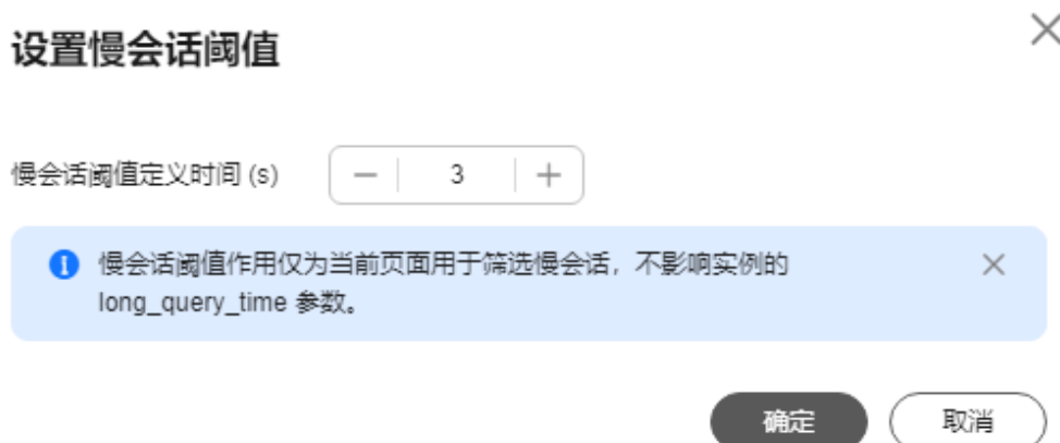
图 3-171 设置慢会话阈值
