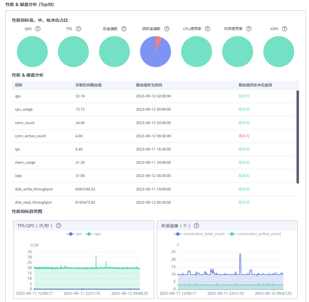
图 3-218 性能&磁盘分析
