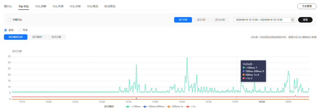
图 7-52 查看特定时间点的 TOP SQL 列表
