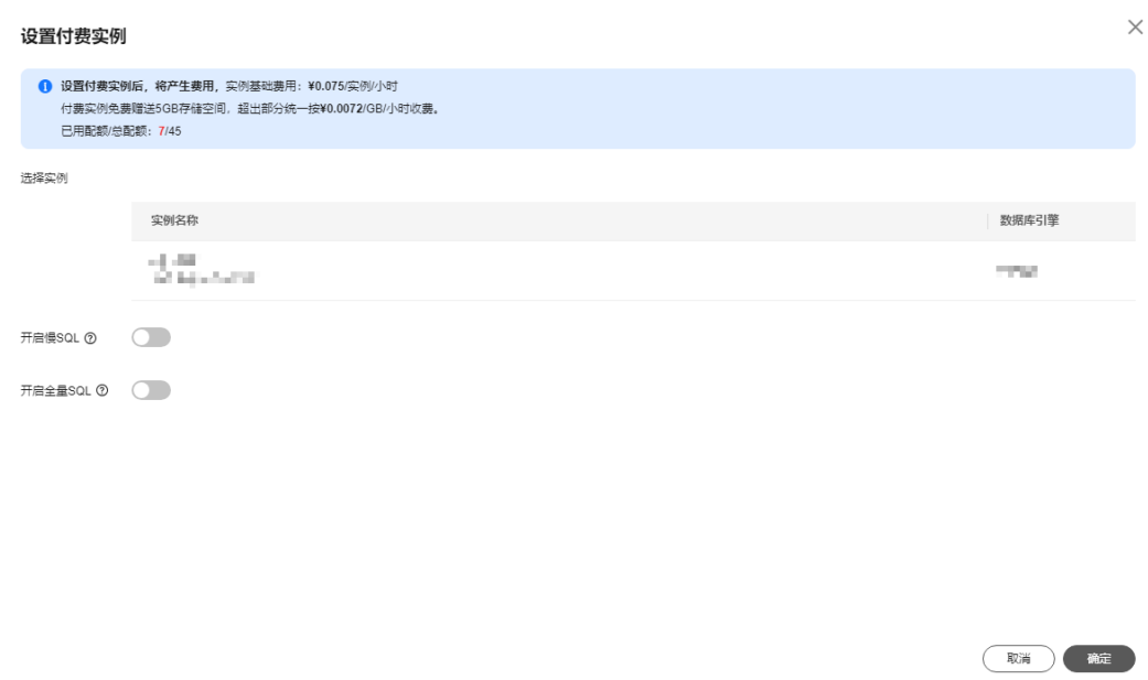
图 3-151 设置付费实例弹窗
