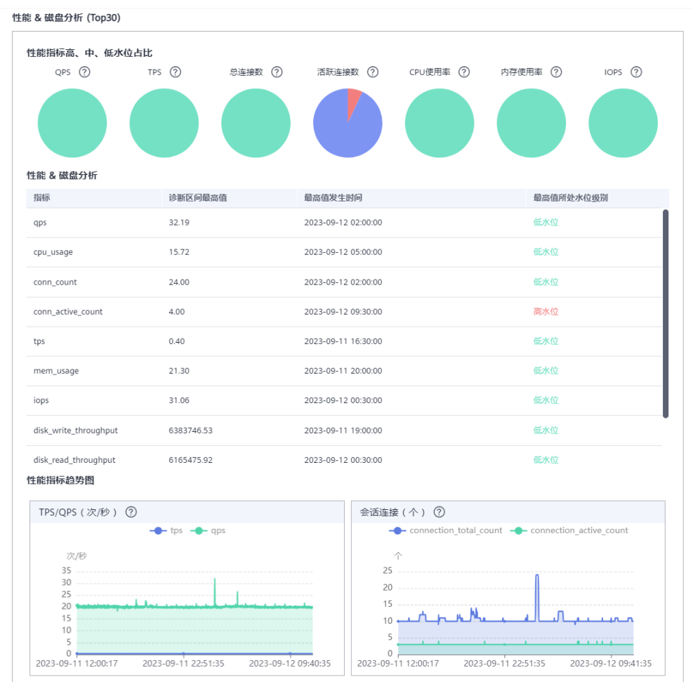
图 6-199 性能&磁盘分析
