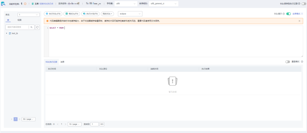
图 3-9 SQL 窗口
