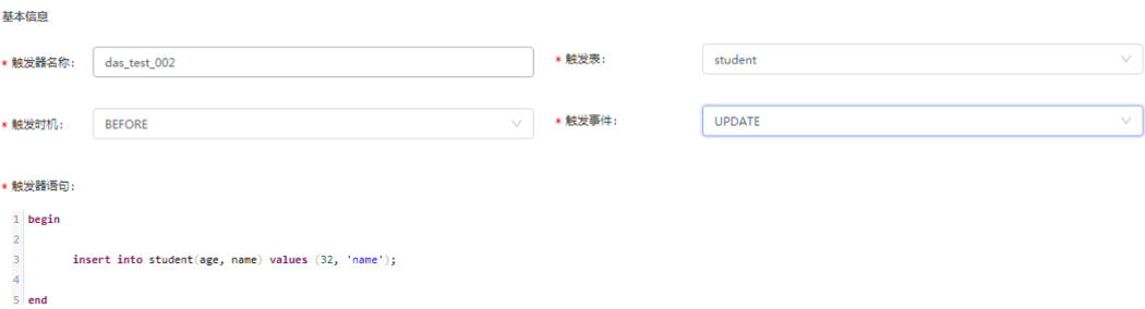
图 6-91 编辑触发器
