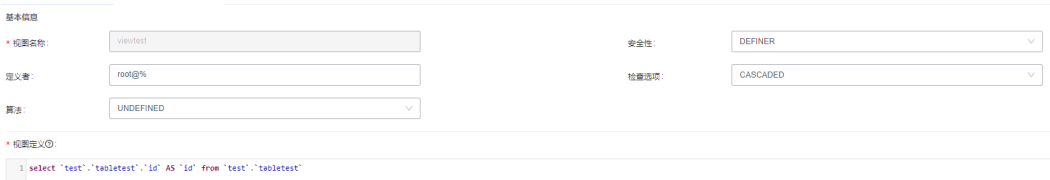
图 6-60 编辑视图
