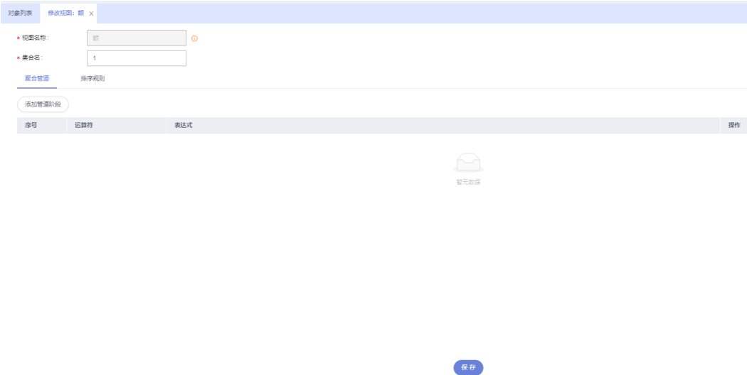
图 11-27 修改视图
