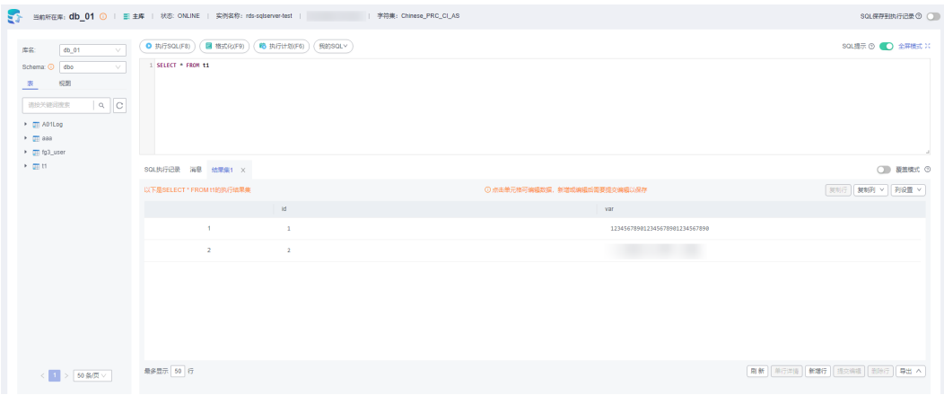
图 4-11 SQL 窗口
