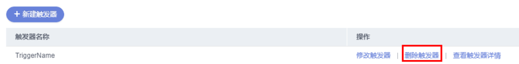
图 4-70 删除触发器
