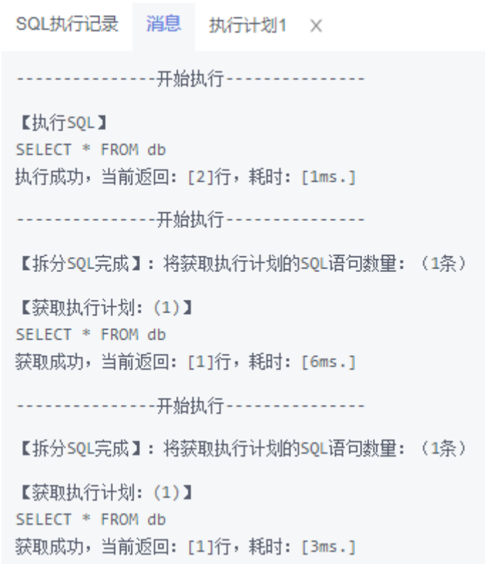
图 6-17 查看消息
