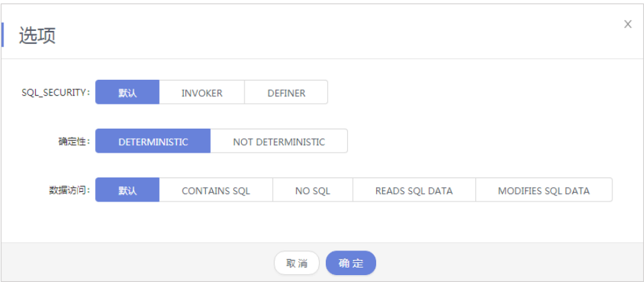
图 8-59 选项界面
