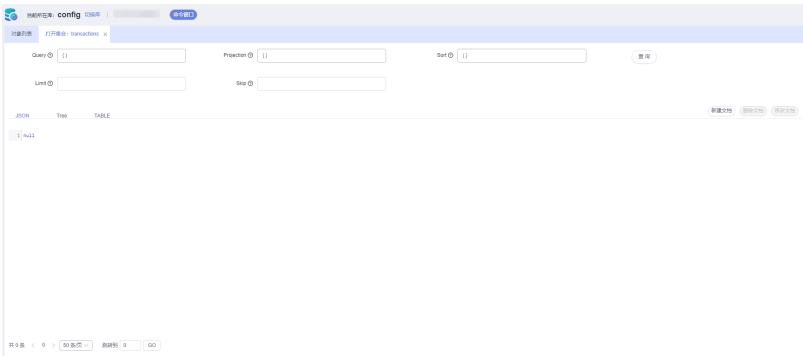
图 11-17 打开集合
