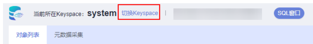
图 9-14 切换 Keyspace
