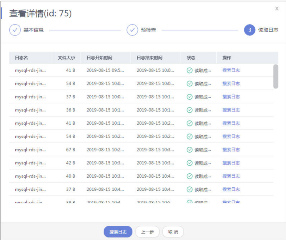
图 3-116 读取日志
