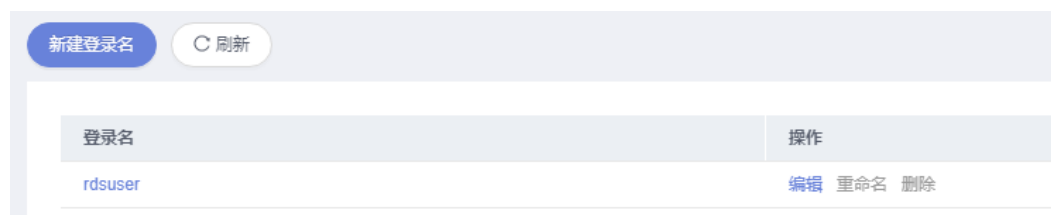
图 4-1 登录名
