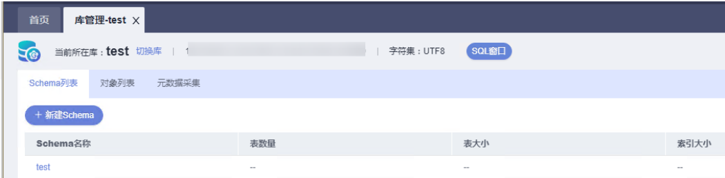
图 7-9 库管理页面
