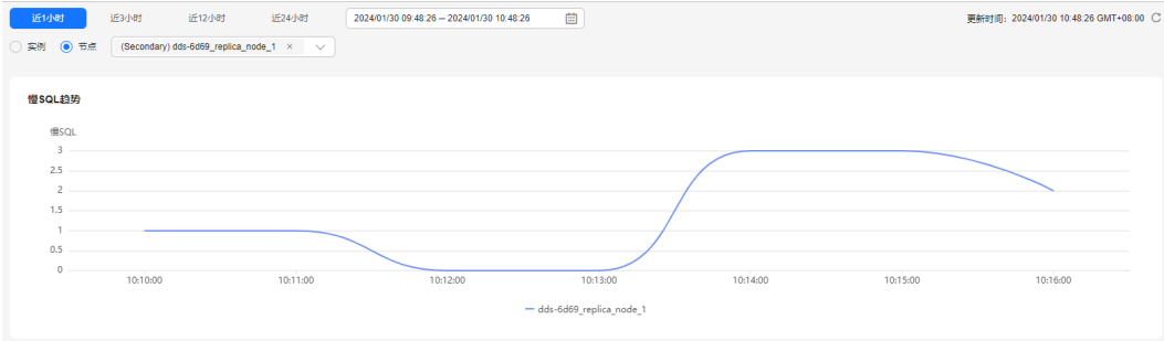
图 11-32 慢 SQL 趋势
