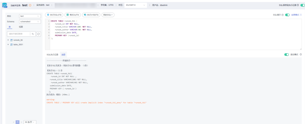
图 10-4 SQL 窗口
