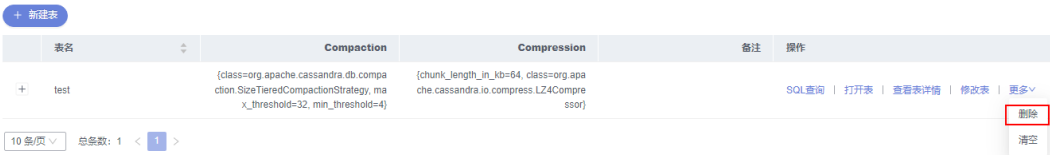
图 9-22 删除表
