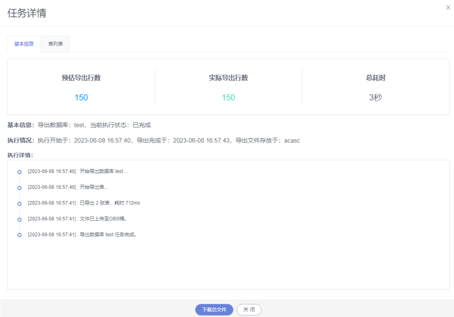
图 5-38 任务详情
