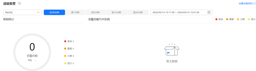
图 5-41 活动告警
