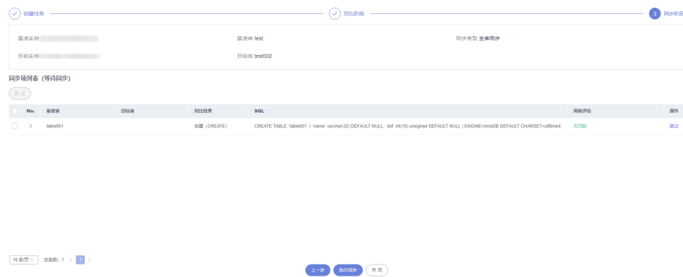
图 6-151 执行同步
