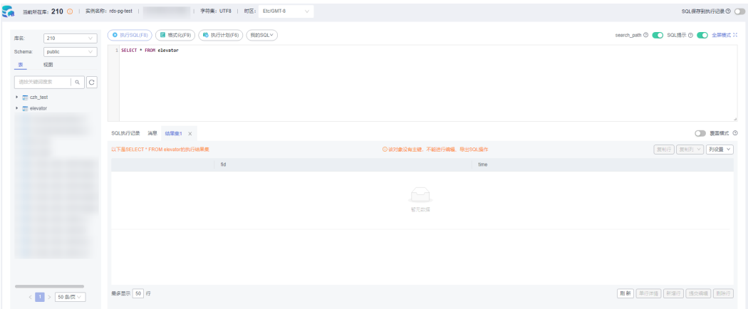
图 5-5 SQL 窗口
