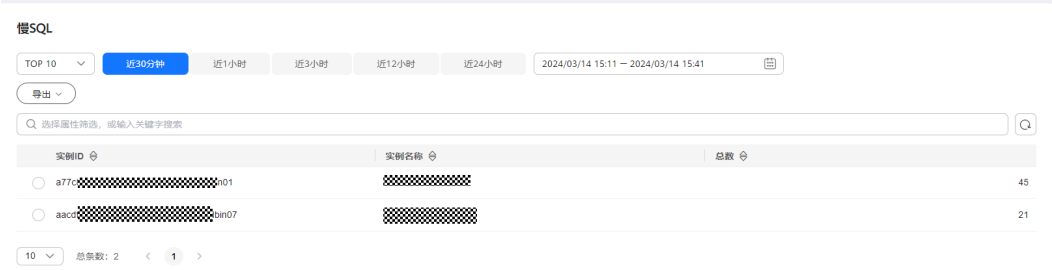
图 5-42 慢 SQL
