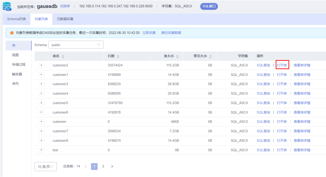
图 10-10 打开表
