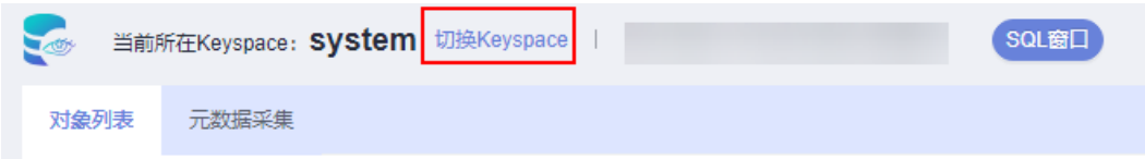
图 9-23 切换 Keyspace
