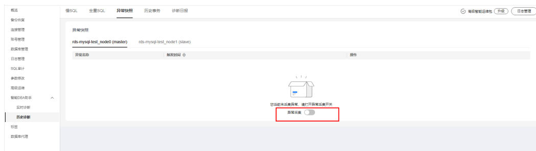
图 3-224 异常快照
