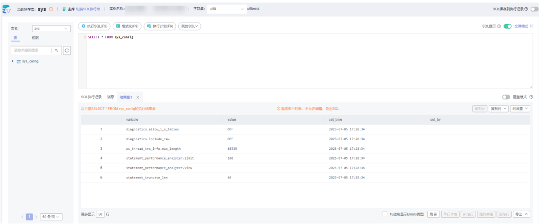
图 8-9 SQL 窗口
