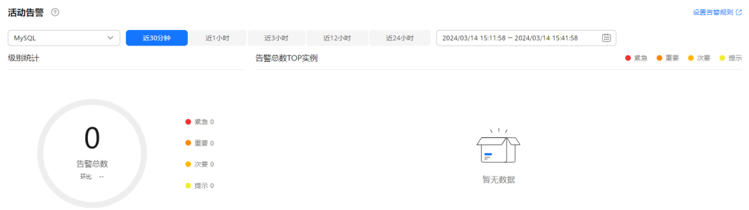
图 8-100 活动告警
