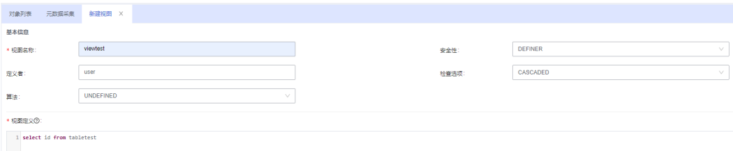
图 6-54 新建视图
