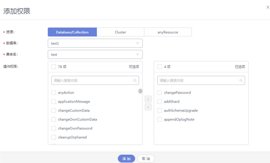
图 11-6 添加权限
