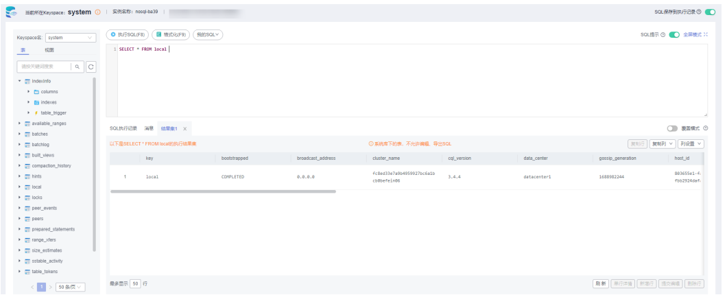
图 9-4 SQL 窗口
