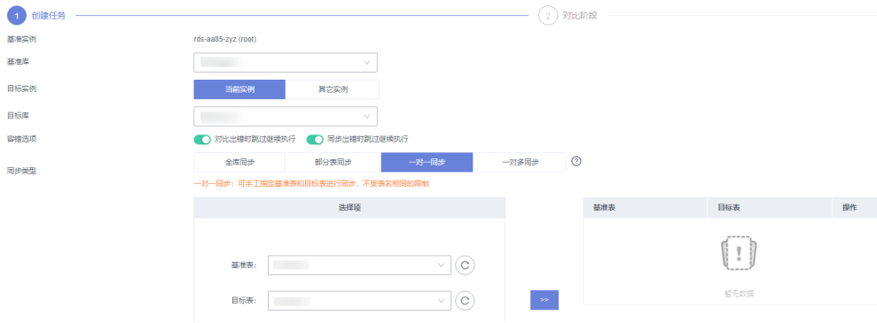
图 3-141 创建任务
