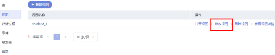
图 3-53 修改视图
