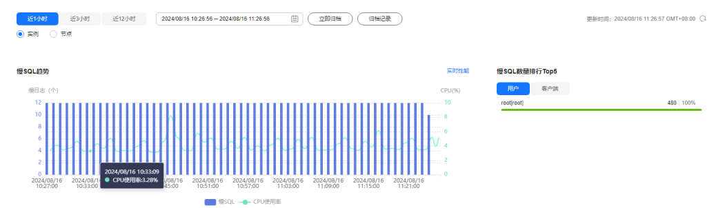
图 5-45 慢日志趋势
