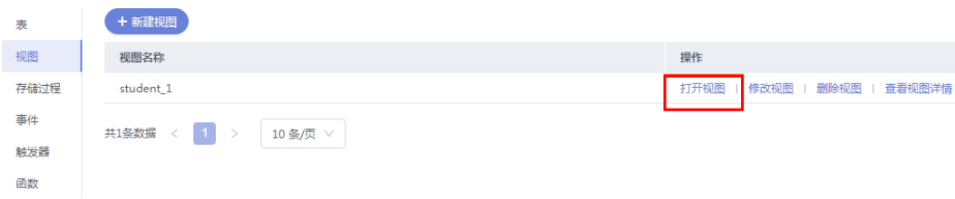
图 8-38 打开视图
