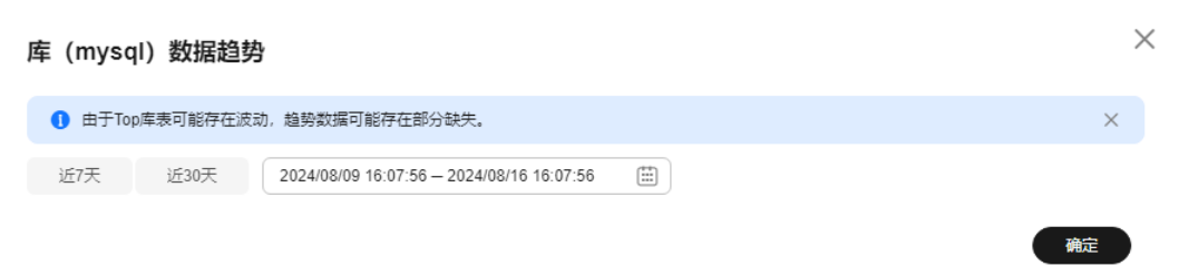
图 3-202 查看趋势
