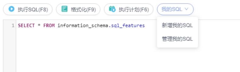
图 7-14 我的 SQL
