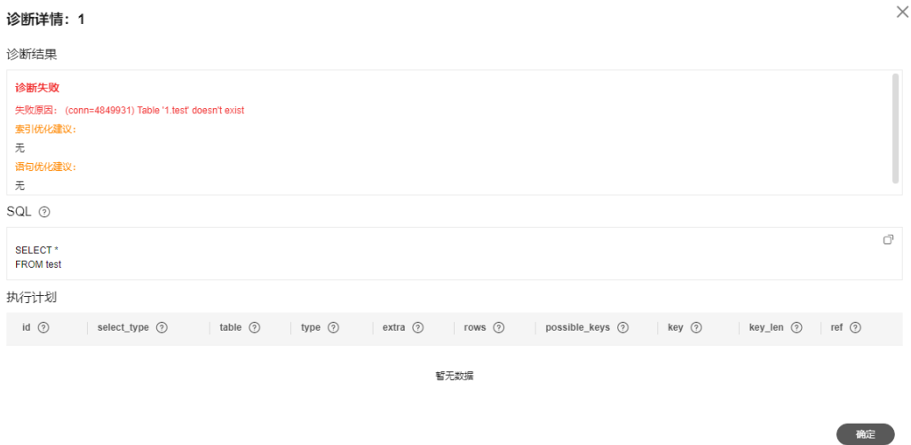
图 3-189 SQL 诊断
