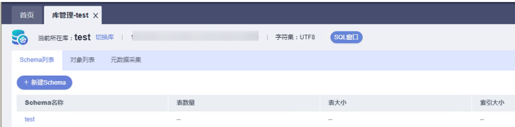
图 7-5 库管理页面
