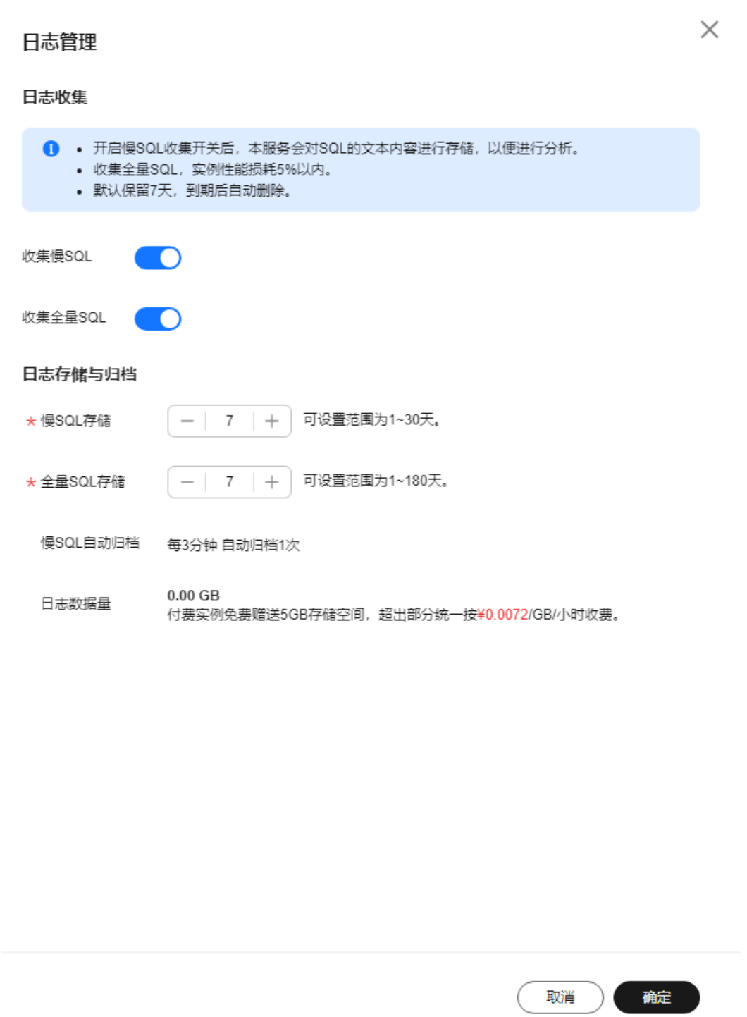
图 3-181 日志管理
