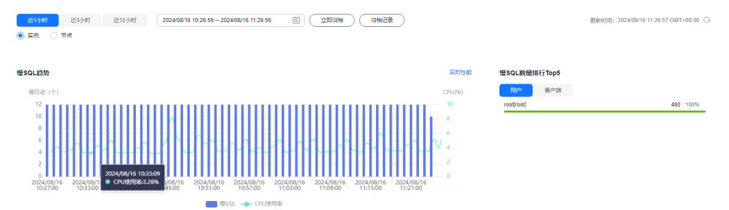
图 8-112 慢日志趋势
