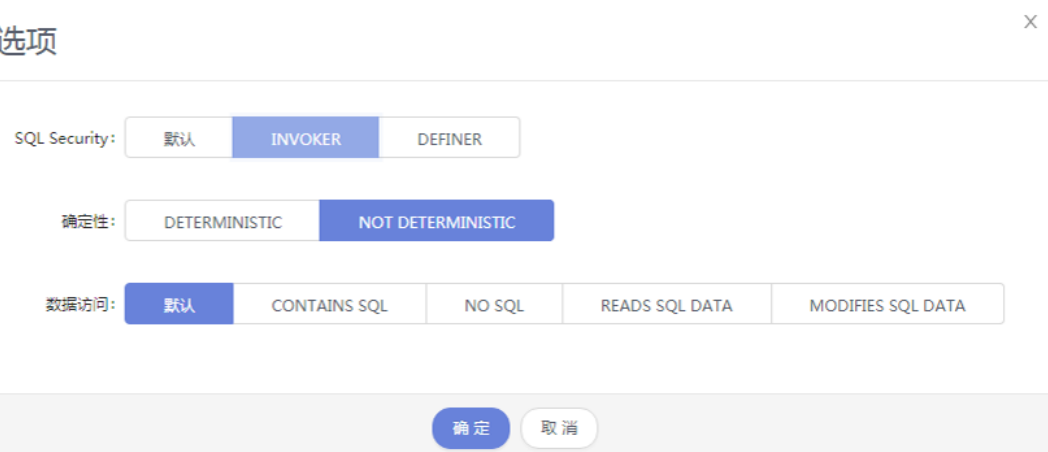
图 8-53 选项界面
