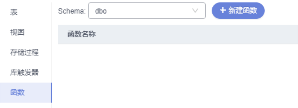
图 4-74 新建函数
