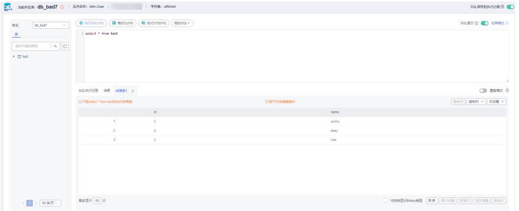
图 12-2 SQL 查询
