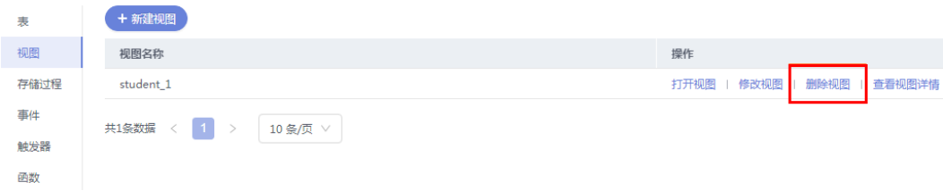
图 3-56 删除视图
