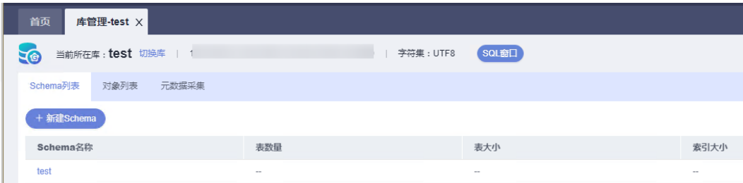
图 7-7 库管理页面
