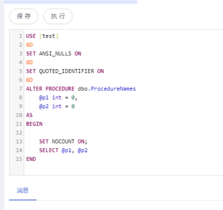
图 4-58 保存修改
