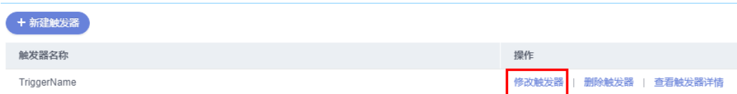
图 4-68 修改触发器
