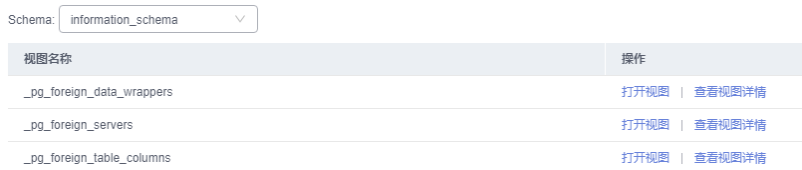
图 7-21 打开视图
