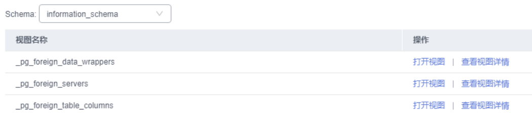
图 10-14 打开视图
