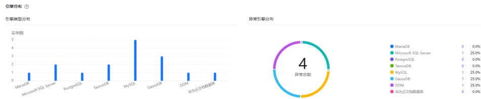
图 5-40 引擎分布
