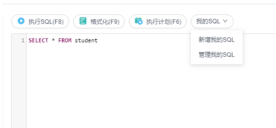
图 12-5 我的 SQL
