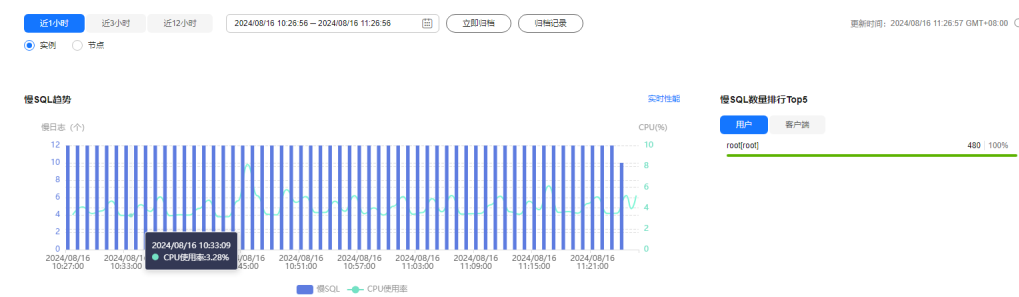
图 6-175 慢日志趋势
