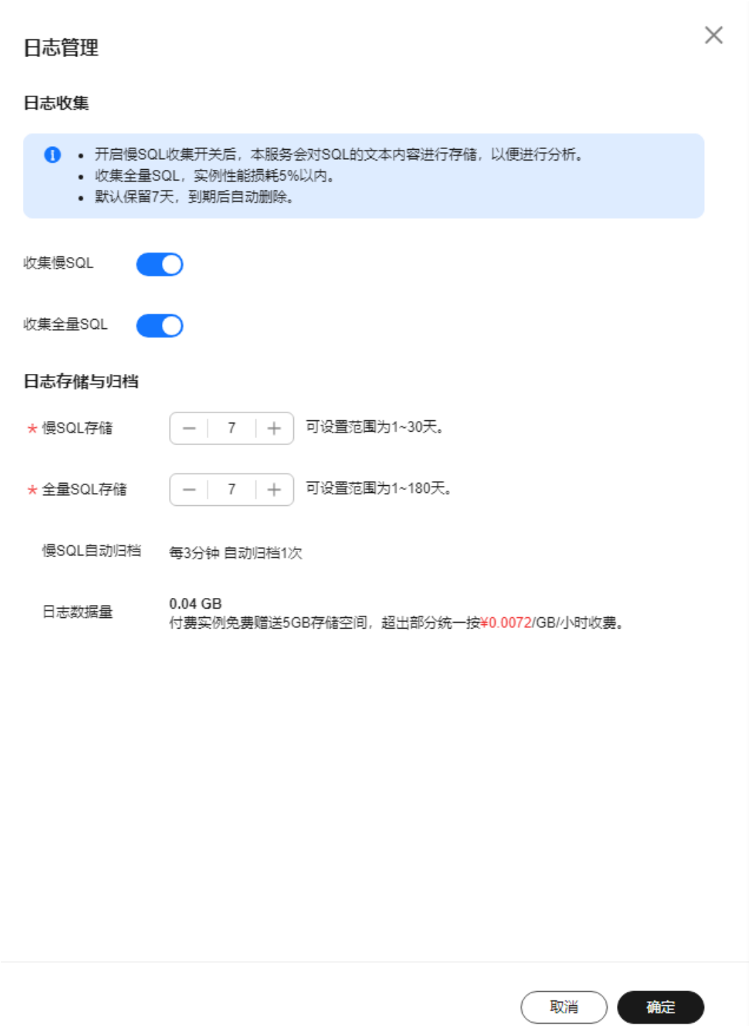
图 3-186 日志管理
