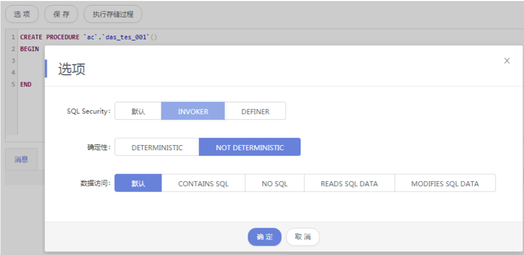
图 6-72 编辑页面
