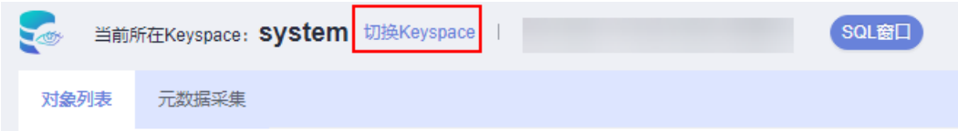
图 9-21 切换 Keyspace
