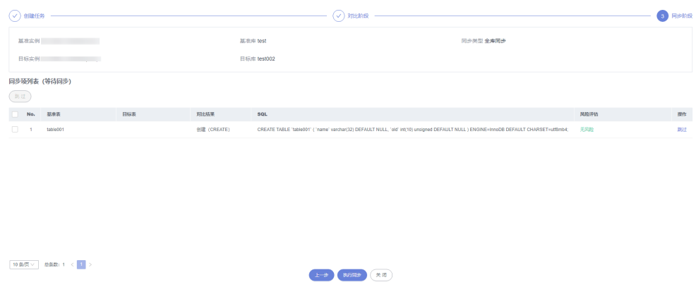
图 3-143 执行同步
