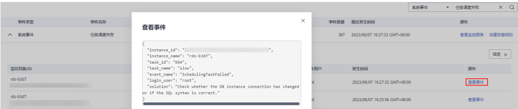
图 14-2 查看事件
