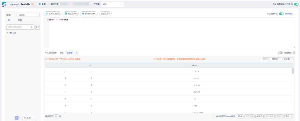
图 6-11 SQL 窗口
