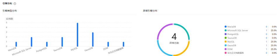
图 8-99 引擎分布
