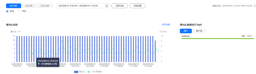
图 3-179 慢日志归档
