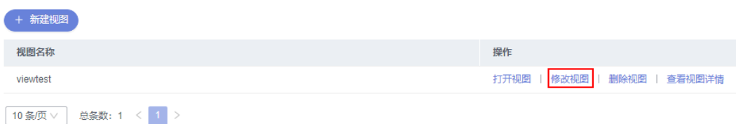
图 6-59 修改视图
