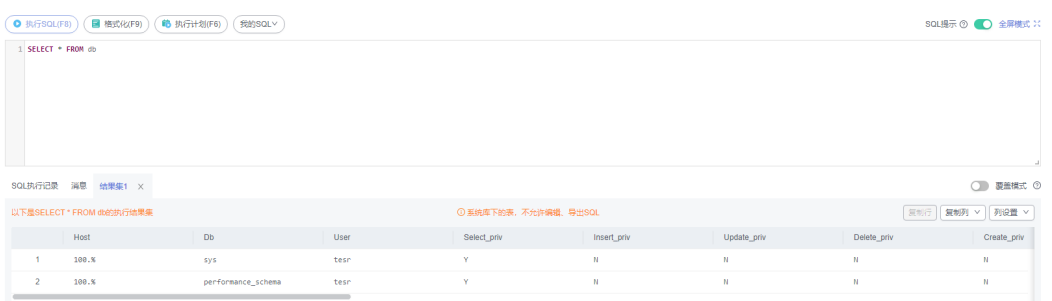
图 5-8 执行 SQL
