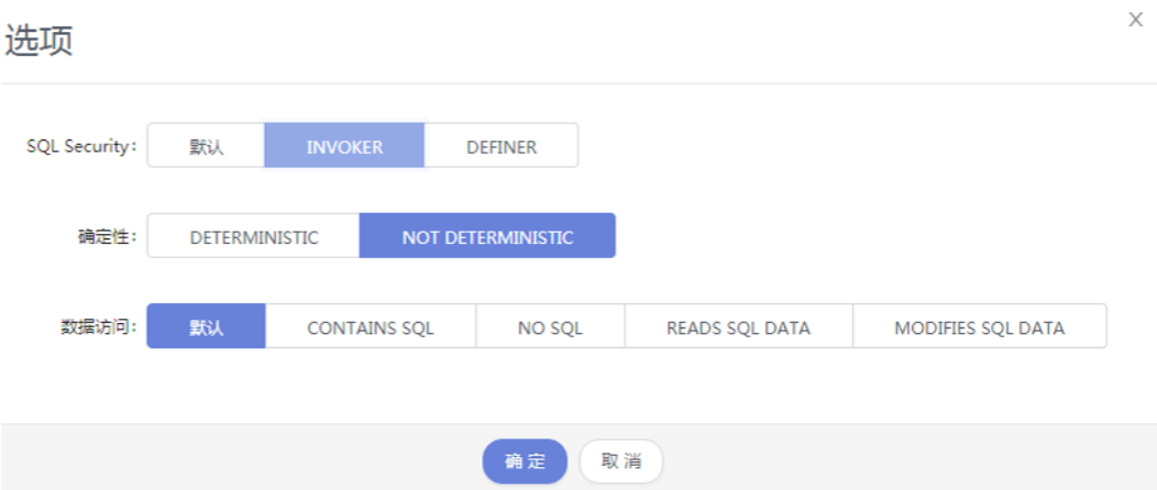
图 8-50 选项界面
