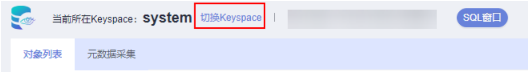
图 9-16 切换 Keyspace
