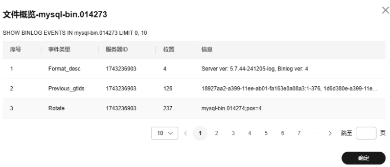
图 3-211 查看概览
