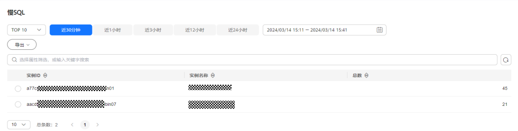
图 8-101 慢 SQL
