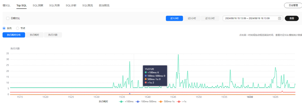
图 12-21 TOP SQL
