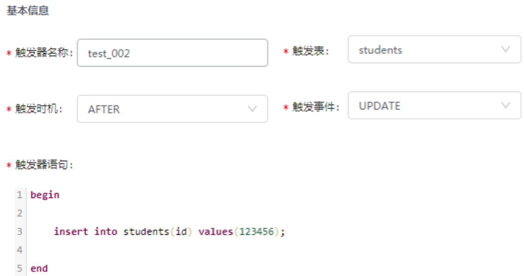
图 6-95 编辑信息
