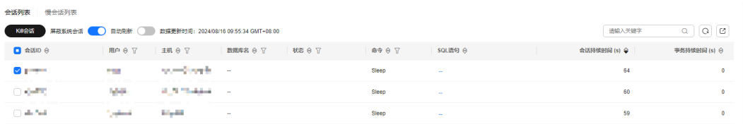
图 8-110 Kill 会话
