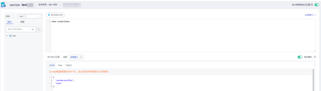
图 11-11 执行命令
