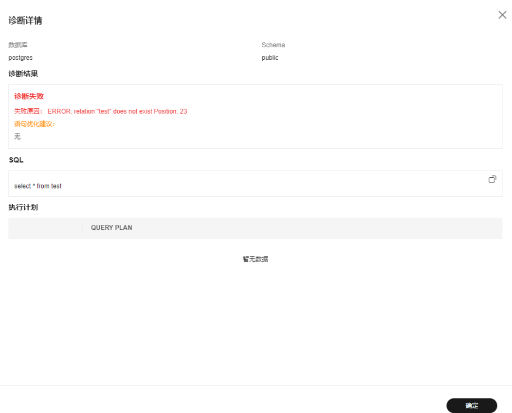
图 5-51 SQL 诊断
