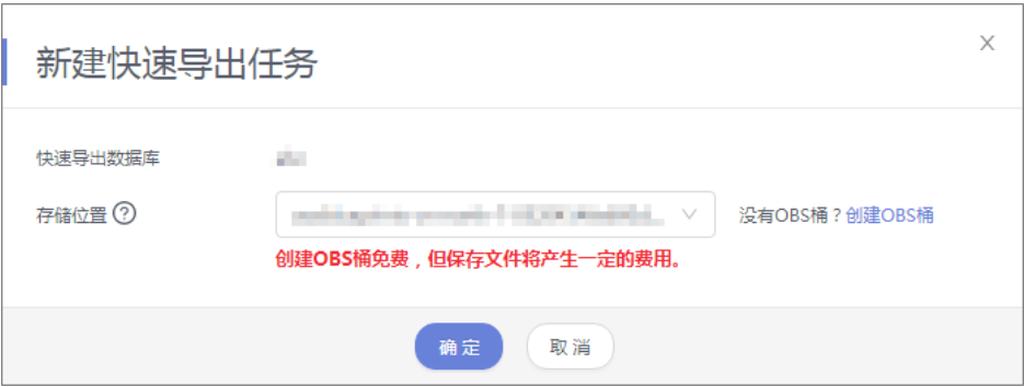
图 9-32 快速导出
