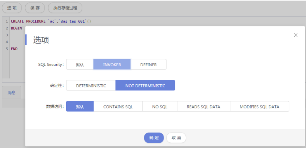
图 6-68 选项页面
