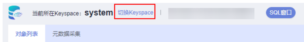
图 9-24 切换 Keyspace
