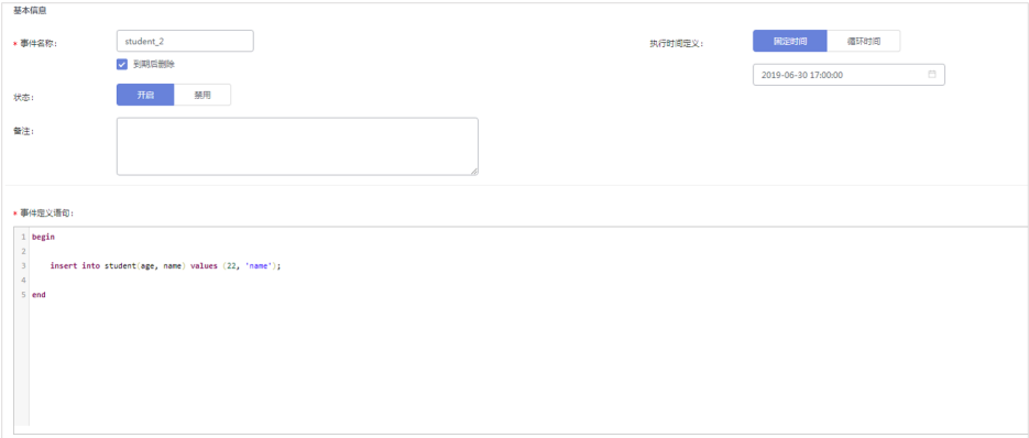
图 6-80 事件详情页
