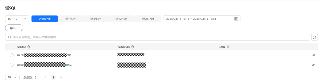
图 6-155 慢 SQL
