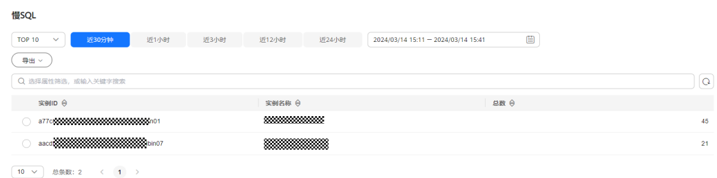
图 3-147 慢 SQL
