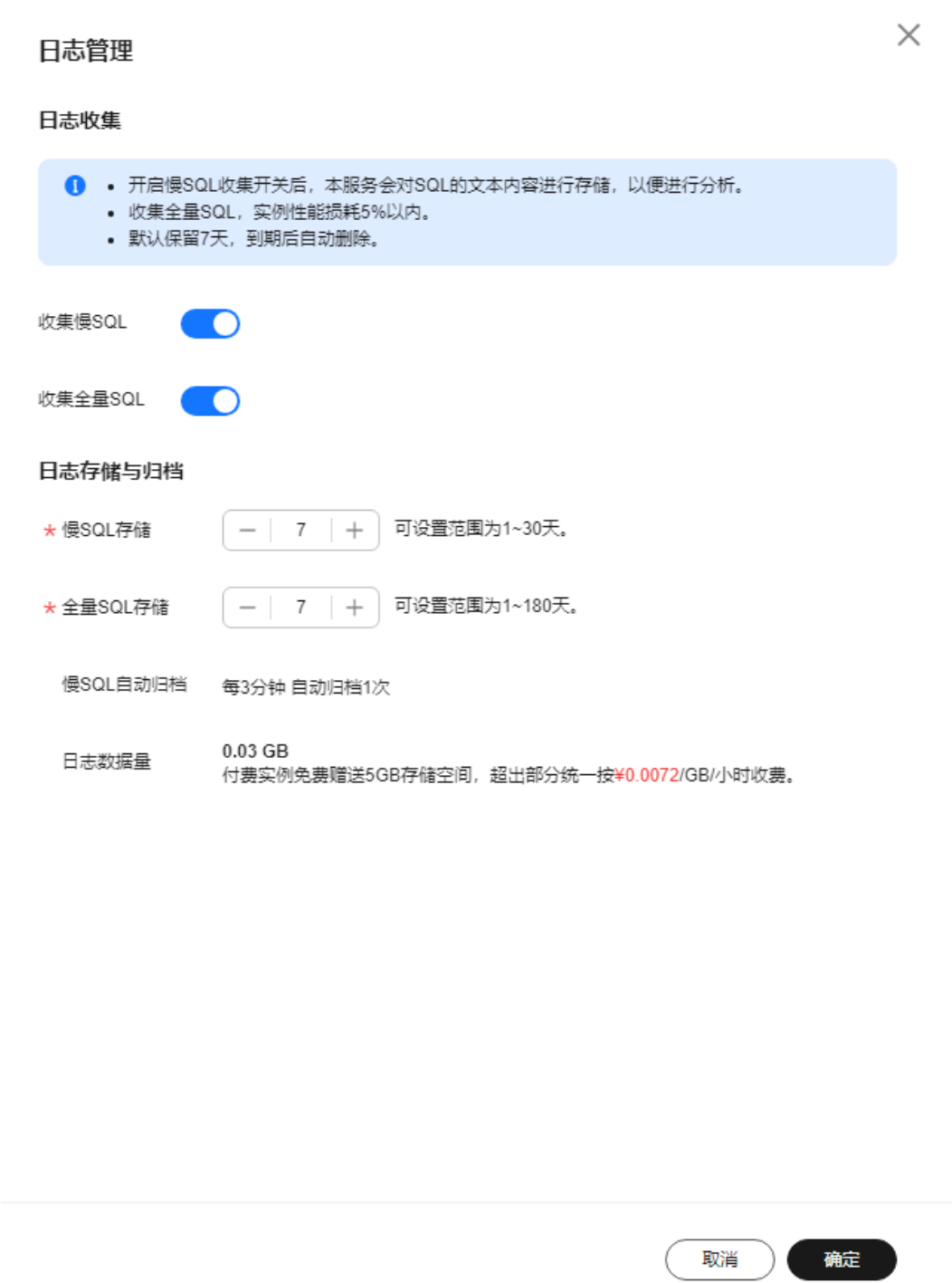
图 7-50 设置慢 SQL 存储时长
