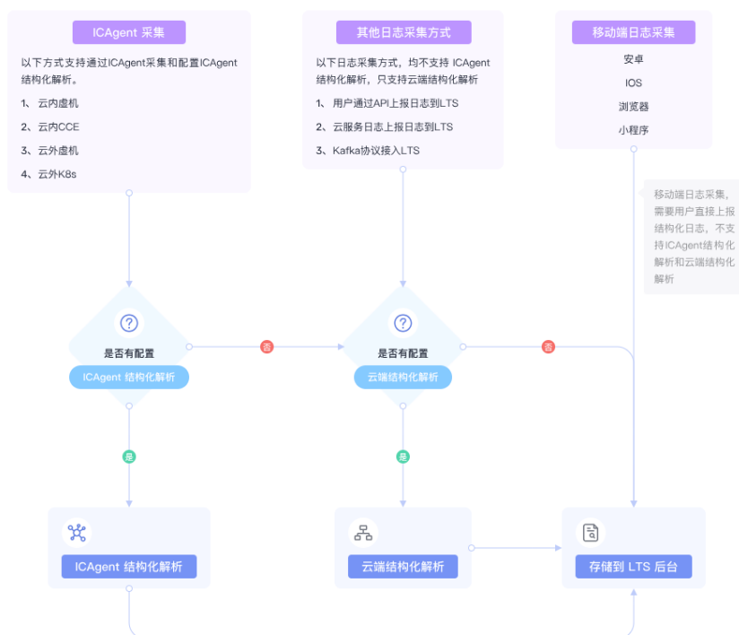
图 6-1 不同解析方式
