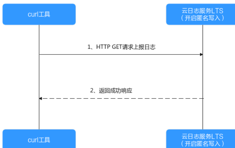
图 4-80 HTTP GET 请求
