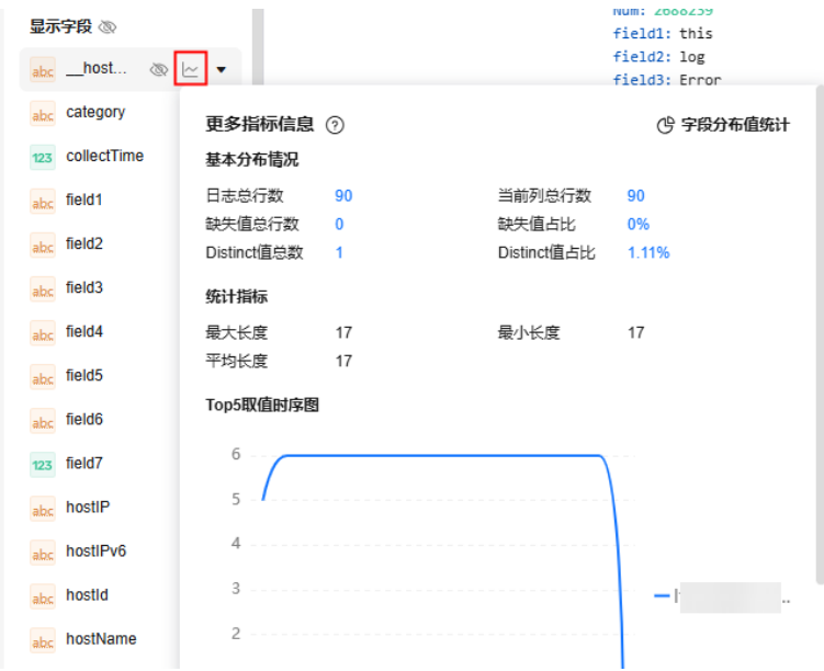
图 6-18 更多指标信息
