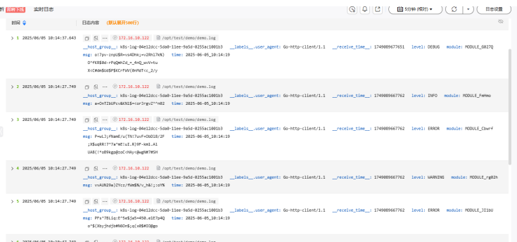
图 4-75 多行-完全正则日志上报结果
