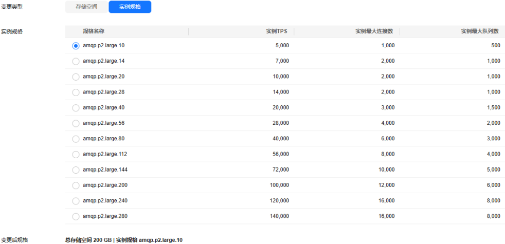
图 9-5 扩容实例规格（RabbitMQ AMQP-0-9-1）
