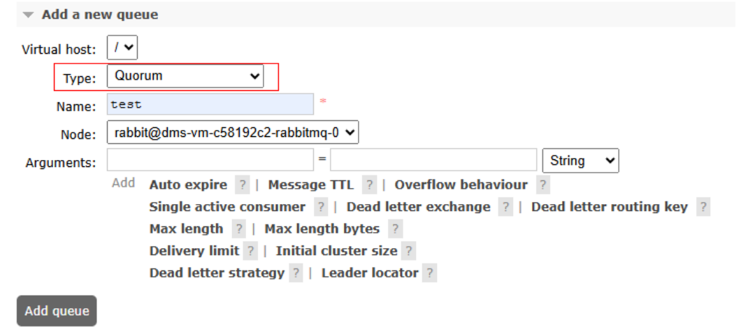
图 4-24 创建仲裁队列
