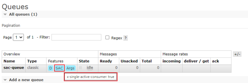
图 4-31 查看队列特性
