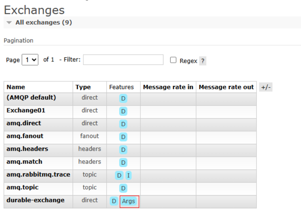
图 7-2 持久化的 Exchange（WebUI）
