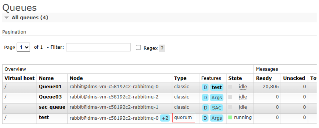
图 4-25 查看队列类型
