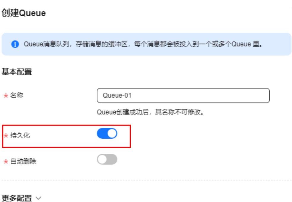
图 7-7 设置 Queue 持久化（控制台）
