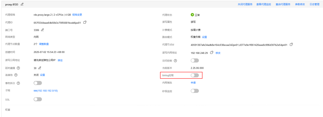
图 13-34 开启 binlog 拉取
