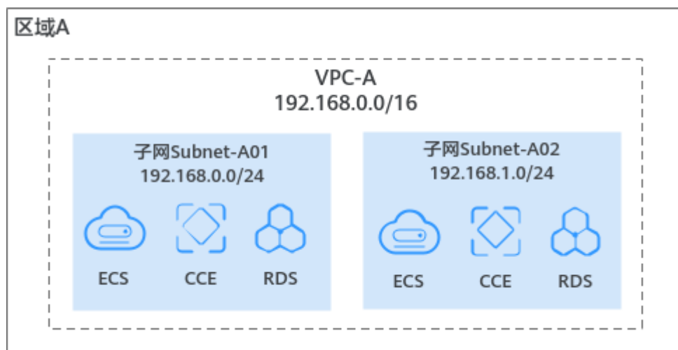
图 2-1 规划 1 个 VPC
