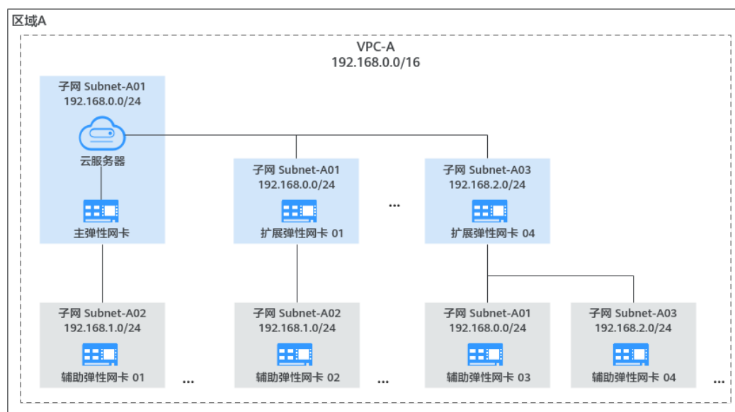
图 5-2 辅助弹性网卡挂载示意图
