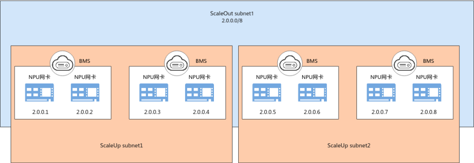
图 14-2 不同子网 NPU 卡间的网络
