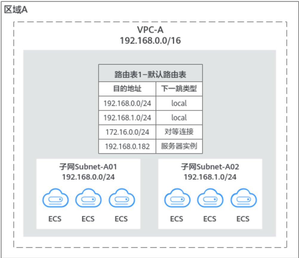
图 2-4 规划一个路由表
