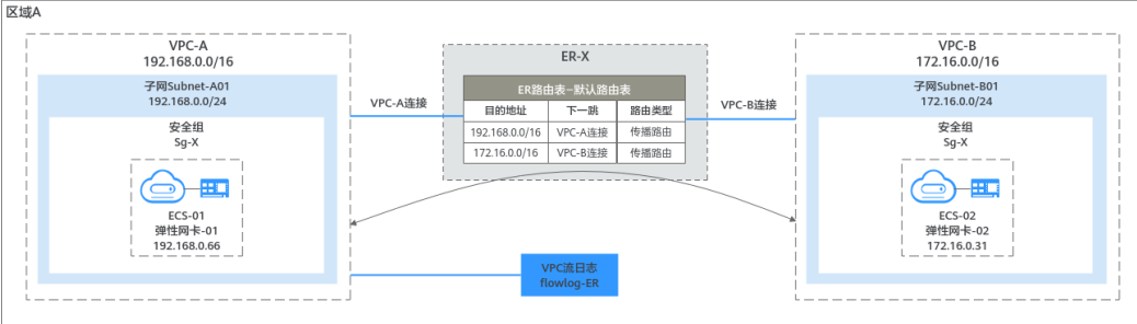
图 12-14 查看不同 VPC 之间的互访流量
