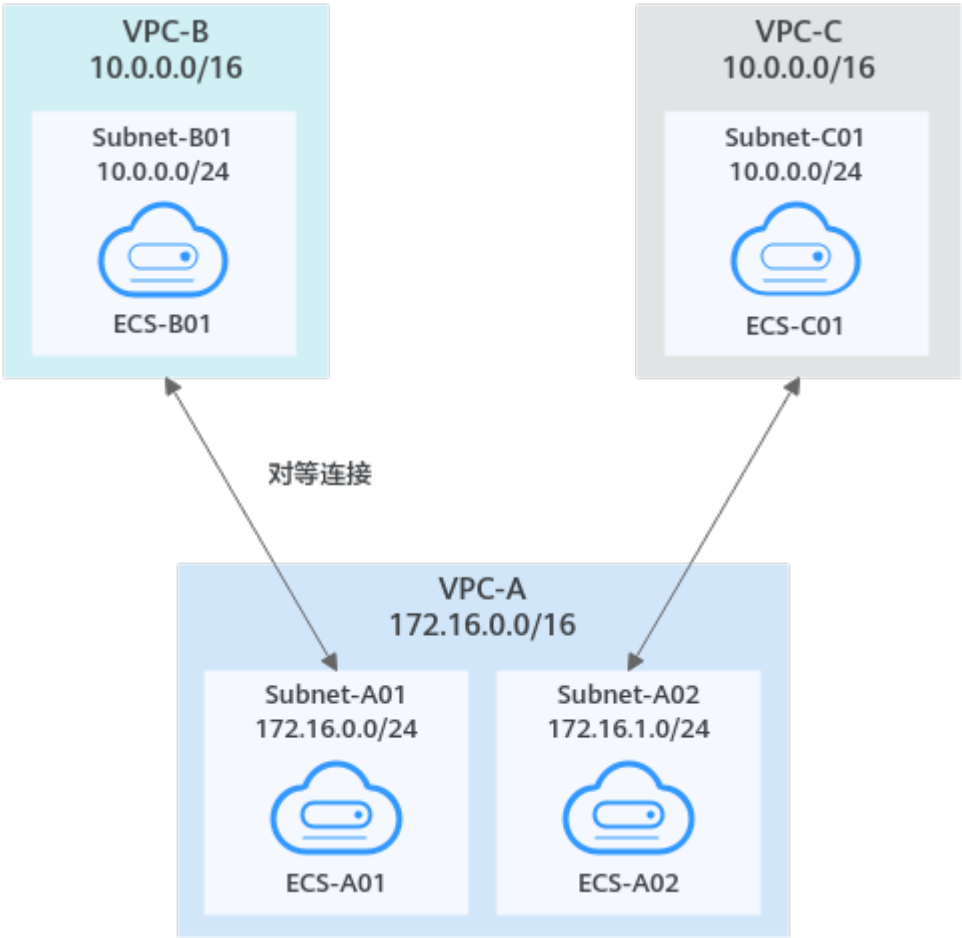
图 8-14 两个 VPC 与一个中心 VPC 的两个子网对等(IPv4)
