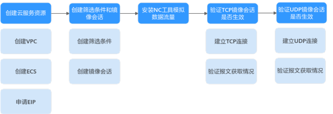
图 13-9 镜像入方向 TCP/UDP 流量
