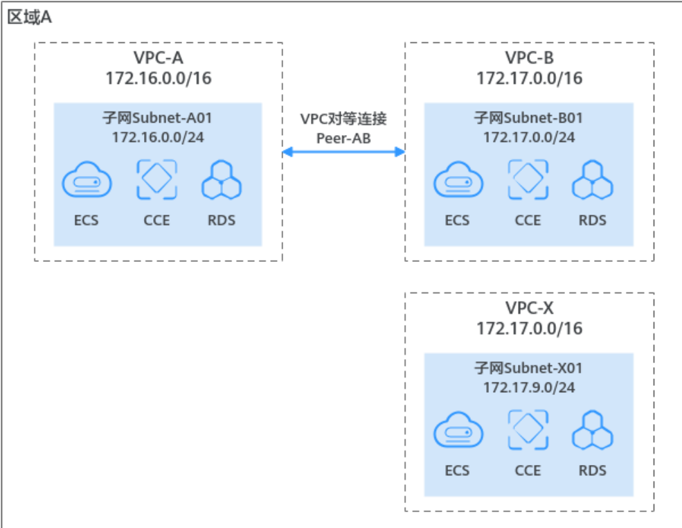
图 2-6 连通同区域的 VPC
