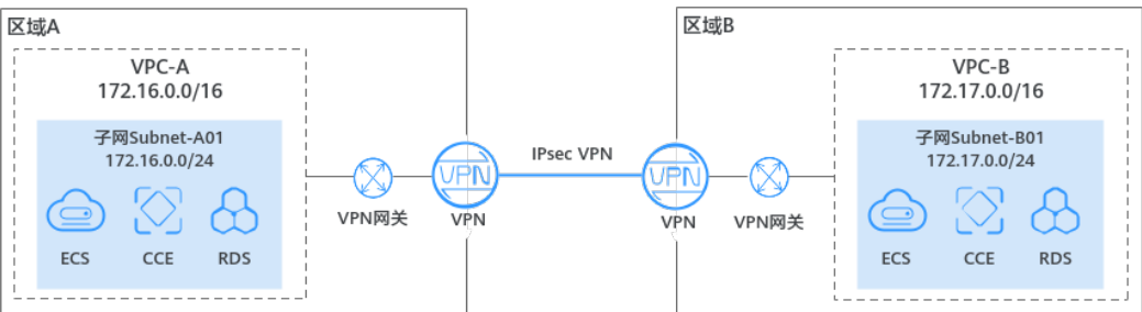
图 2-13 通过 VPN 连通不同区域 VPC
