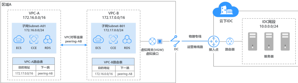
图 2-22 通过对等连接连通同区域的多个 VPC 和云下 IDC 的网络
