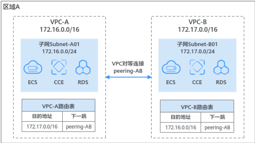
图 3-3 通过对等连接连通同区域 VPC
