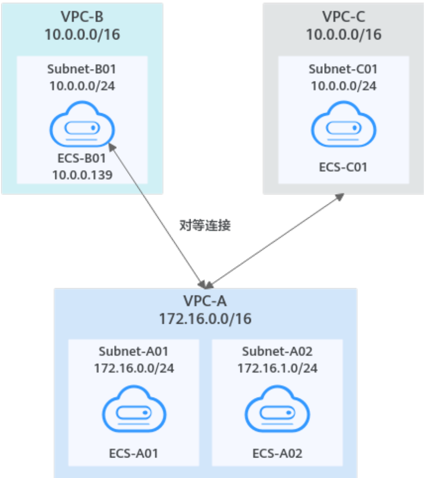
图 8-19 一个中心 VPC 通过最长匹配原则与两个 VPC 对等(IPv4)
