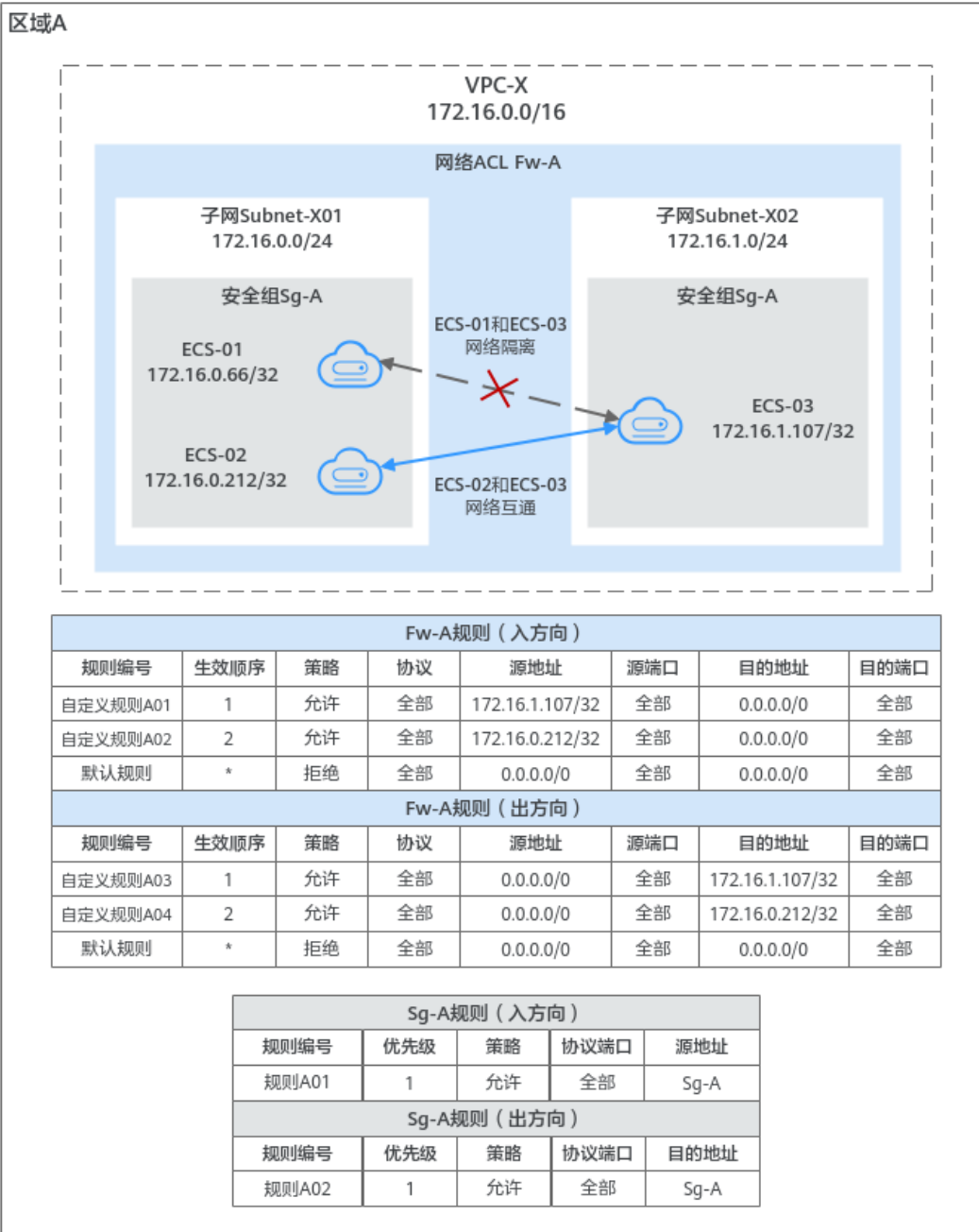
图 6-34 控制不同子网内实例的互通和隔离
