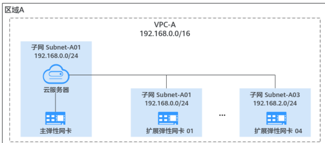
图 5-1 弹性网卡挂载示意图
