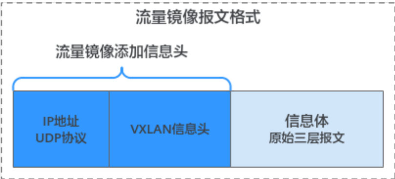
图 13-4 流量镜像报文格式
