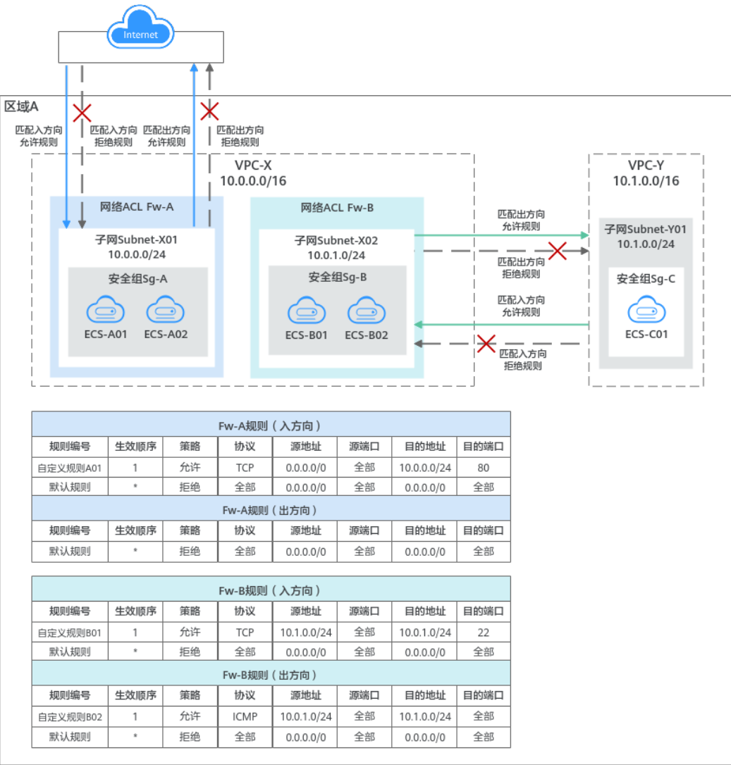
图 6-31 网络 ACL 架构图
