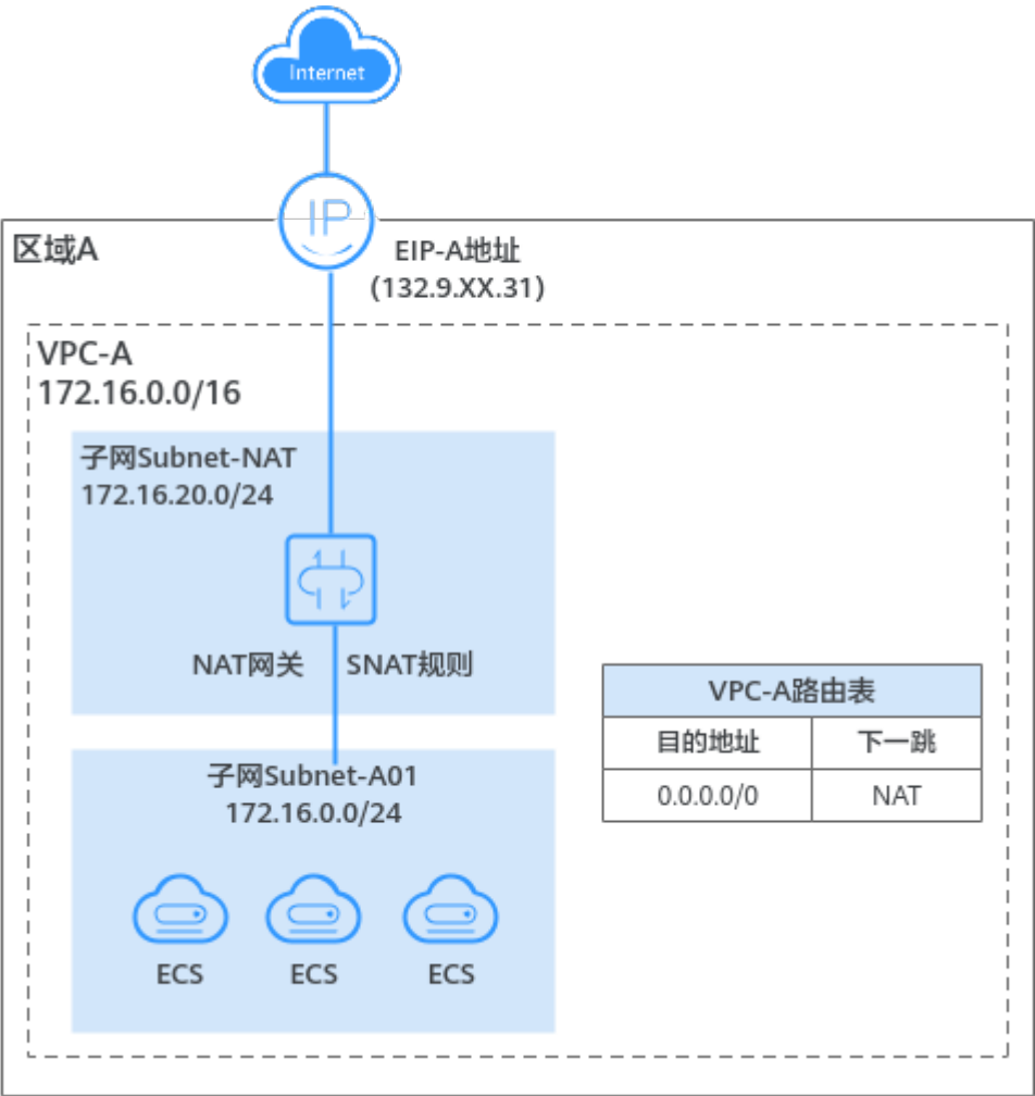
图 3-5 通过 NAT 网关实现 VPC 内 ECS 访问公网
