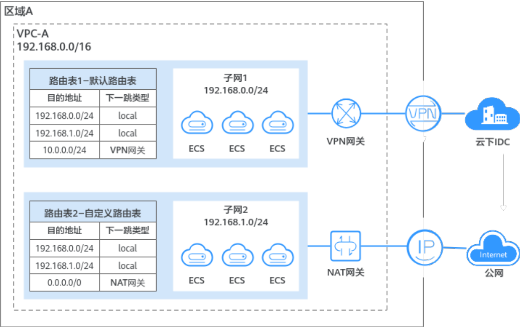
图 3-2 子网关联默认路由表和自定义路由
