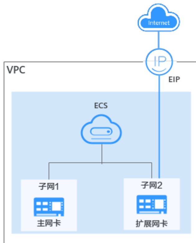
图 5-3 通过 ECS 扩展网卡访问公网的组网示意图
