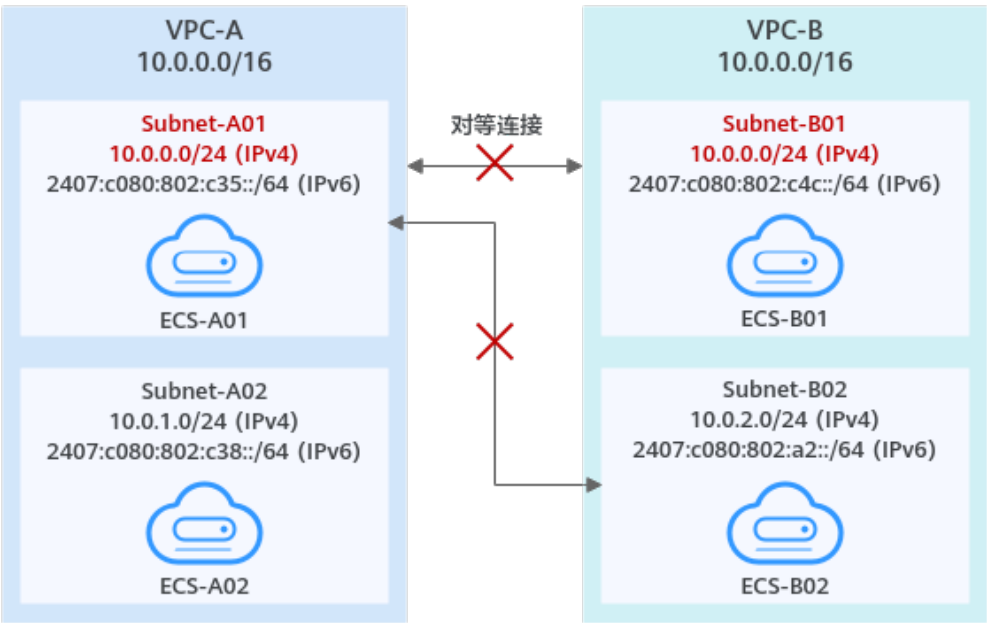
图 8-24 VPC 网段重叠，且部分子网重叠(IPv6)
