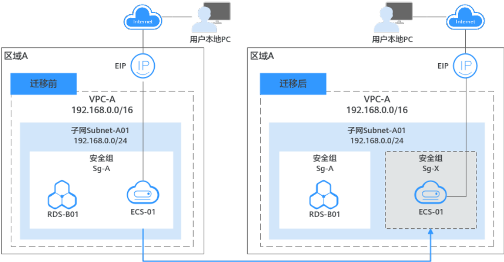
图 6-27 将 ECS 从多业务实例共用安全组迁移至独立安全组
