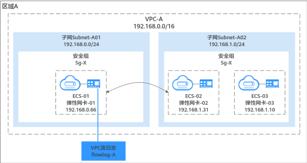
图 13-8 镜像入方向 TCP/UDP 流量
