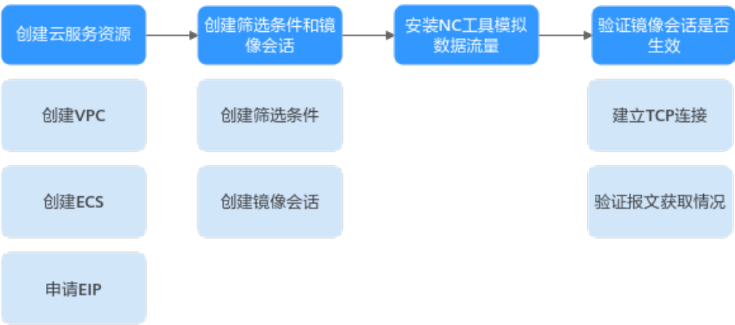
图 13-7 镜像入方向 TCP 流量
