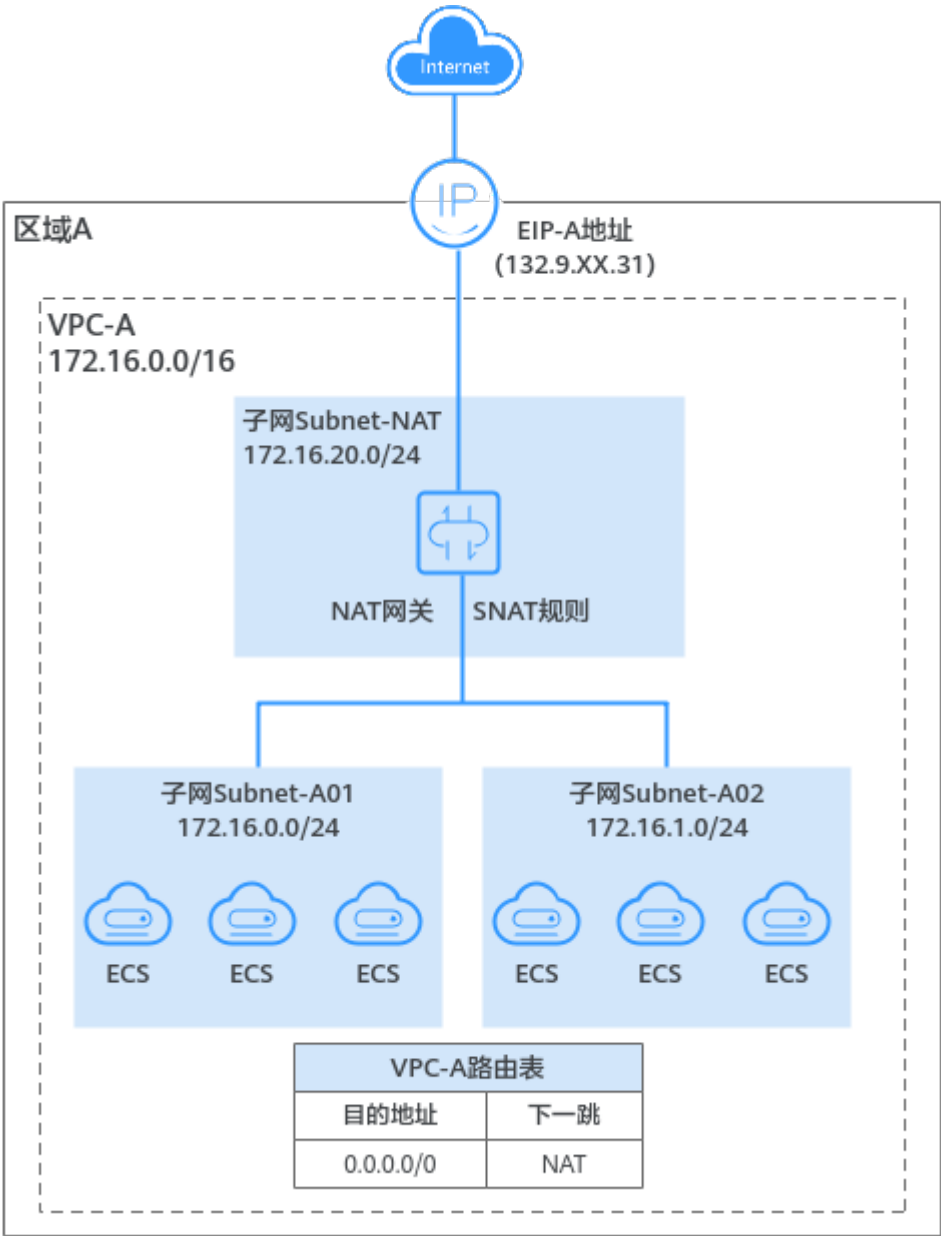
图 2-16 通过 NAT 网关实现 VPC 内 ECS 访问公网（同一个 VPC 内的 ECS 共用 EIP）
