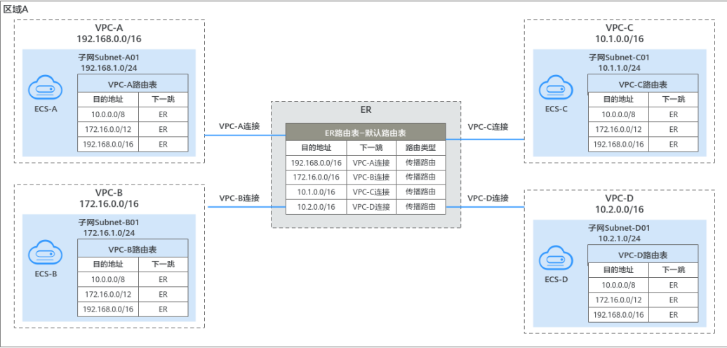
图 3-4 通过企业路由器连通同区域 VPC
