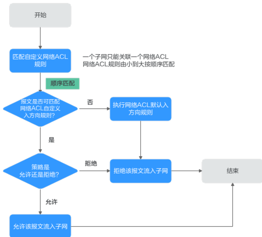
图 6-32 网络 ACL 匹配顺序
