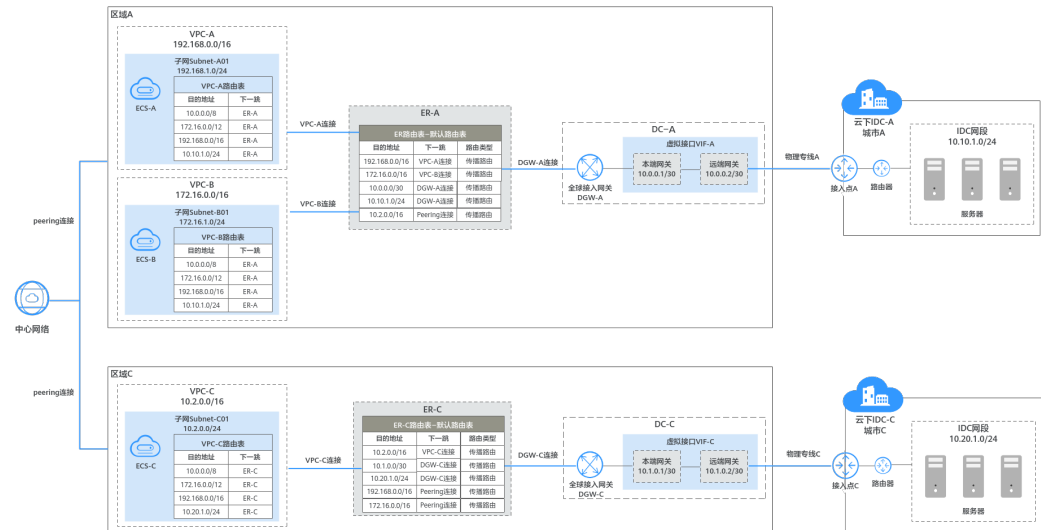
图 2-25 通过中心网络连通不同区域的多个 VPC 和云下 IDC
