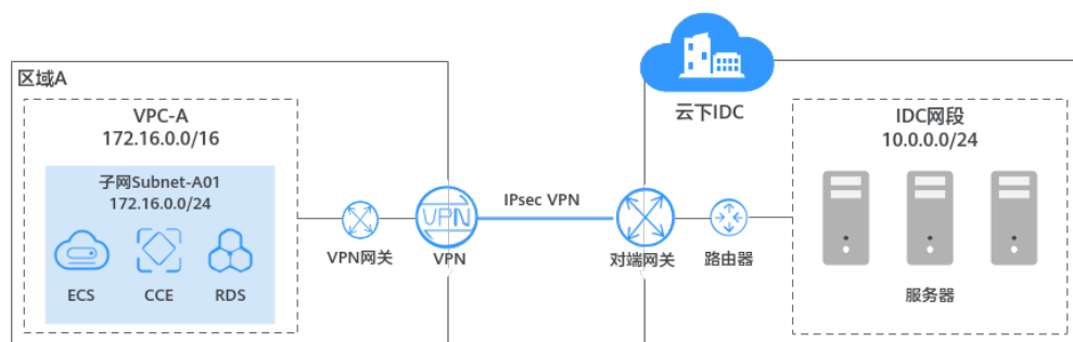
图 2-20 通过 VPN 连通 VPC 和云下 IDC
