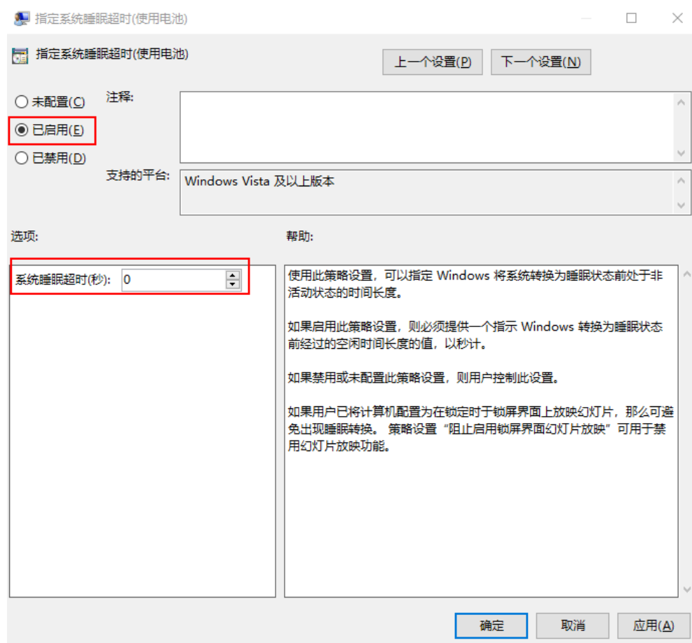
图 15-29 指定系统睡眠超时（使用电池）
