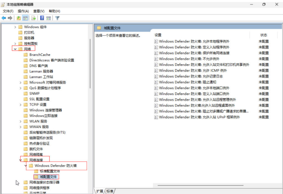
图 15-6 域配置文件列表
