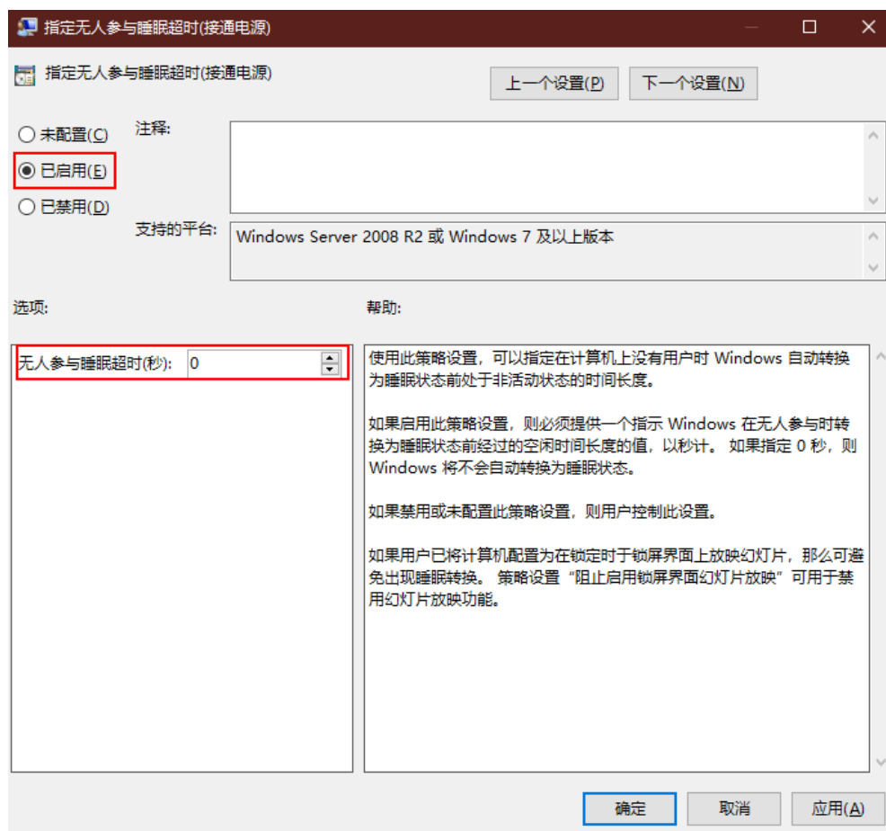
图 15-31 指定无人参与睡眠超时（接通电源）
