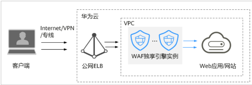
图 3-10 独享模式部署架构（独享引擎实例后端未部署内网 ELB）
