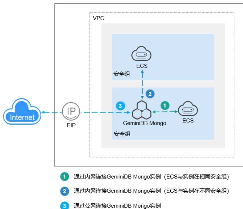
图 3-1 通过内网和公网连接实例
