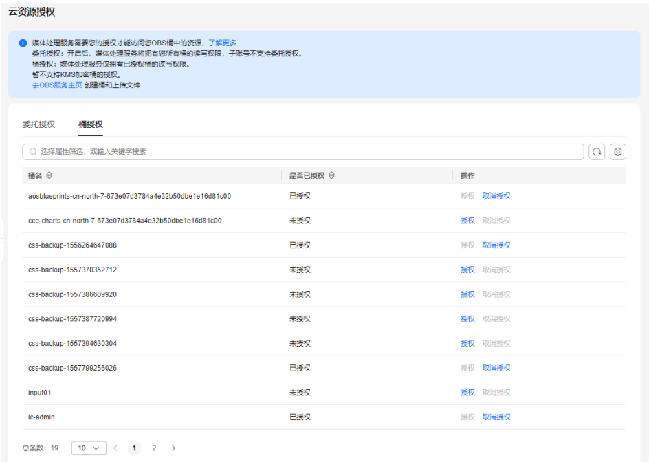
图 4-4 云资源授权
