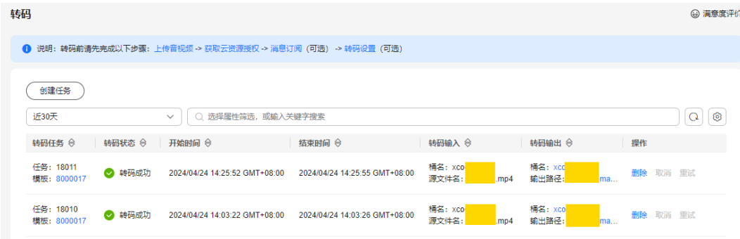
图 4-2 转码任务
