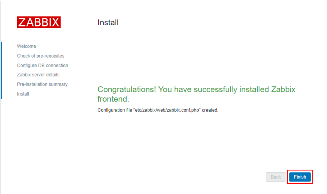
图 3-23 初始化完成
