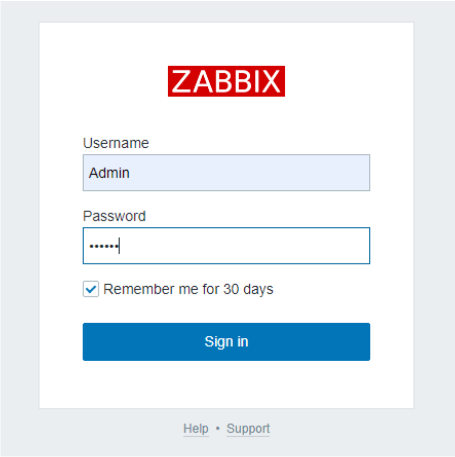
图 3-24 登录 Zabbix
