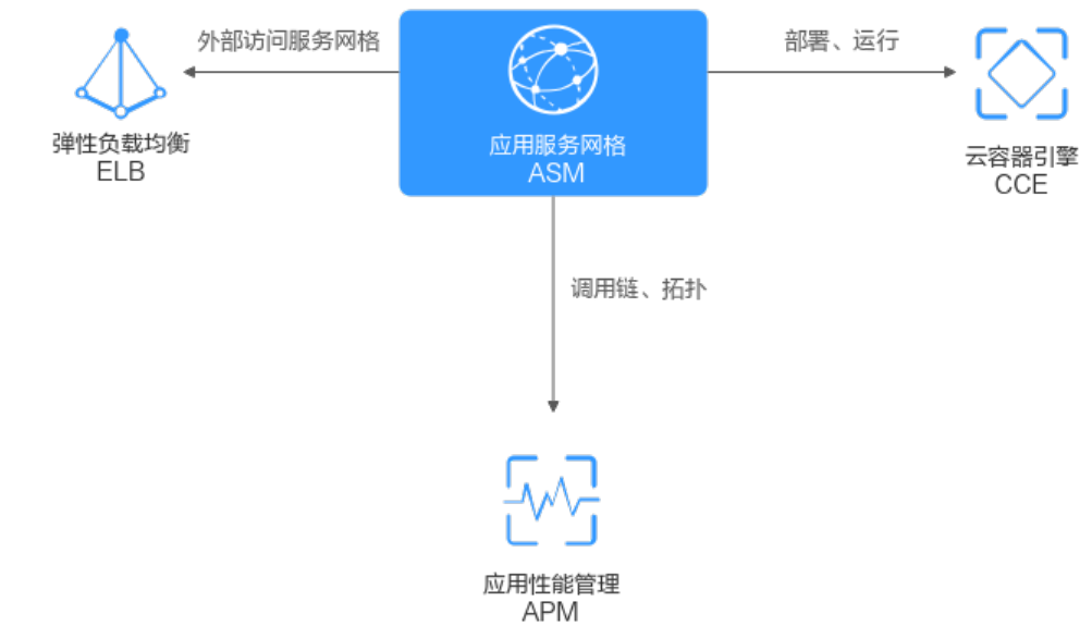
图 10-1 应用服务网格与其他云服务关系
