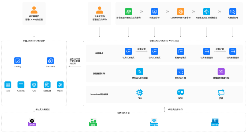
图 1-1 产品架构图
