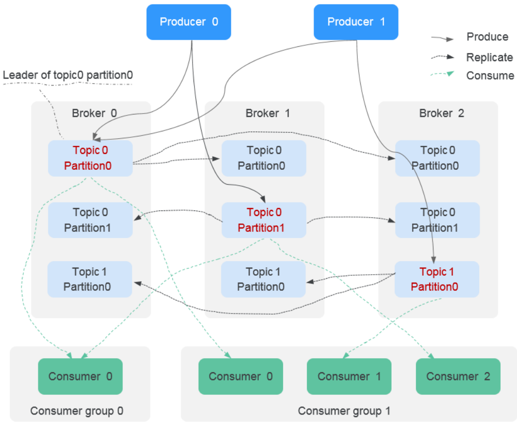
图 11-1 Kafka 消息流
