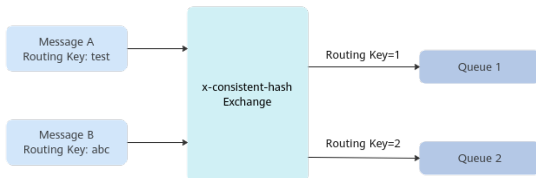
图 12-6 x-consistent-hash Exchange 示例
