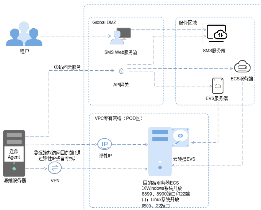
图 12-1 主机迁移服务网络示意图
