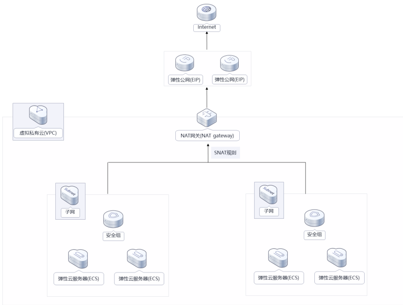
图 1-1 方案架构
