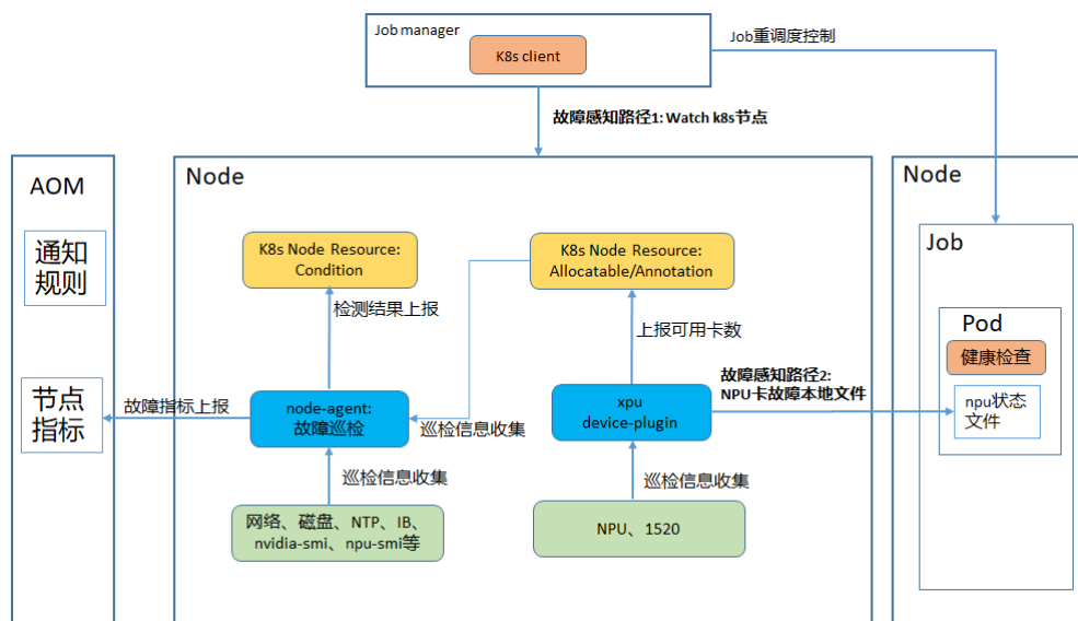
图 10-13 节点故障上报
