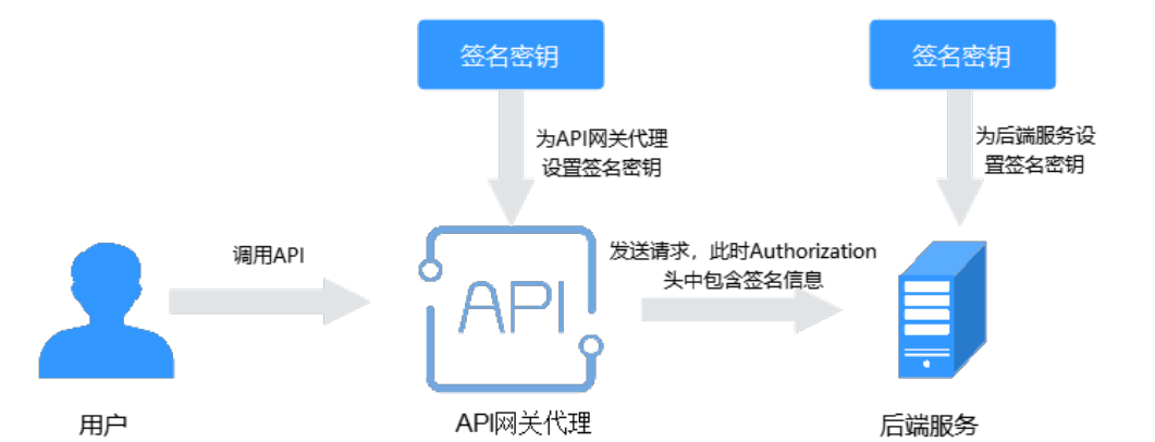
图 5-7 签名密钥流程图
