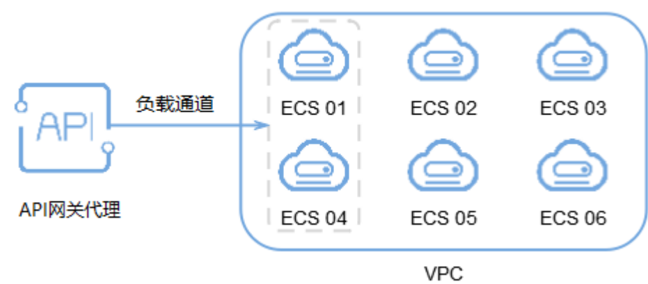
图 5-8 通过 API 网关代理访问负载通道中的 ECS
