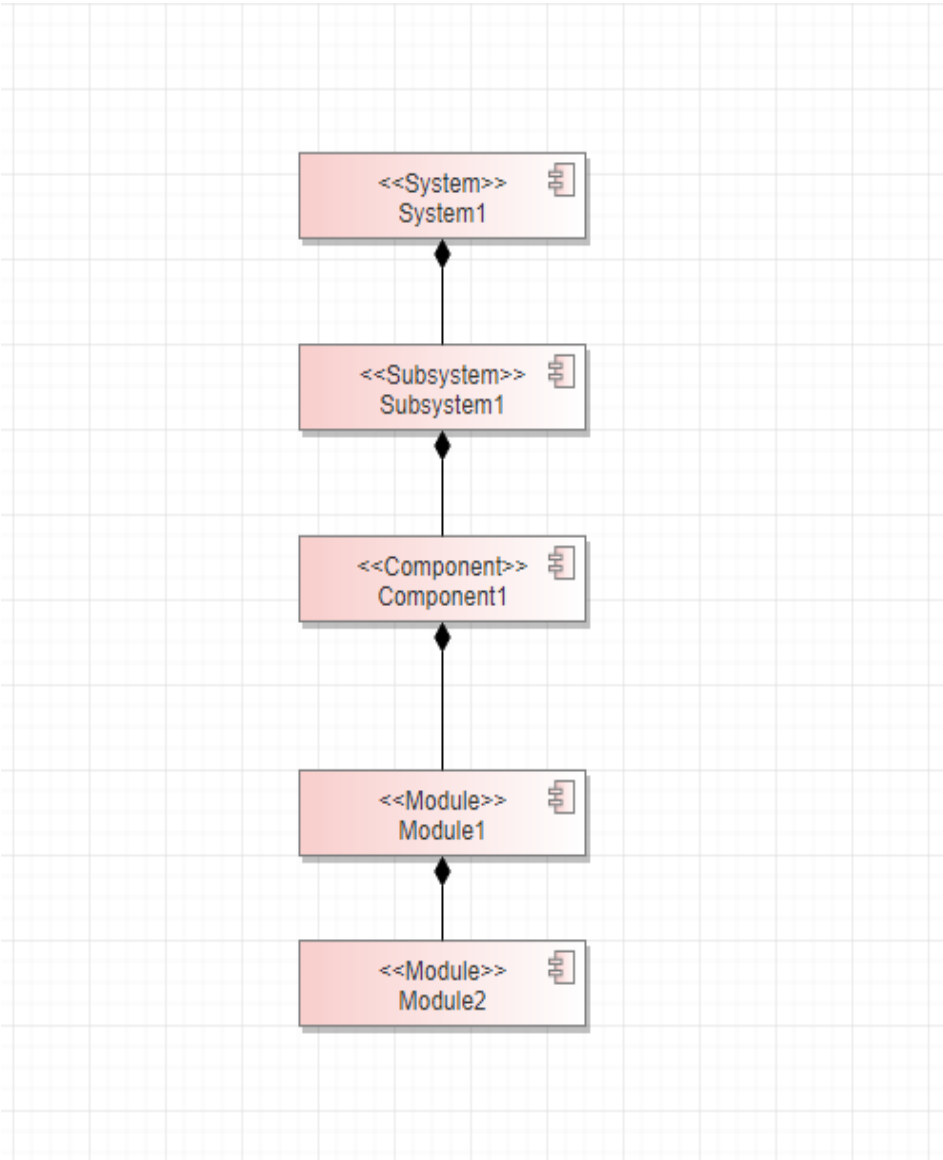
架构信息树展示结果：
