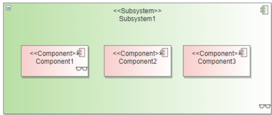
2层逻辑模型。
