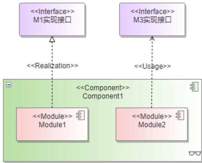
2层逻辑模型。
