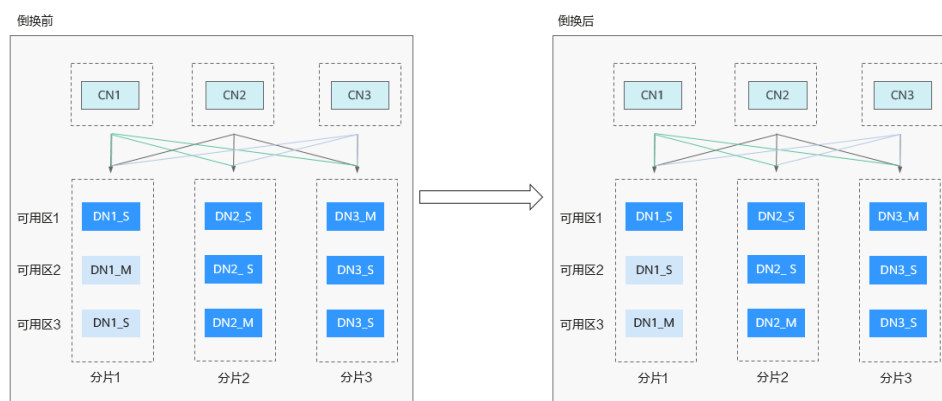
图 8-42 DN 主备倒换示意图
