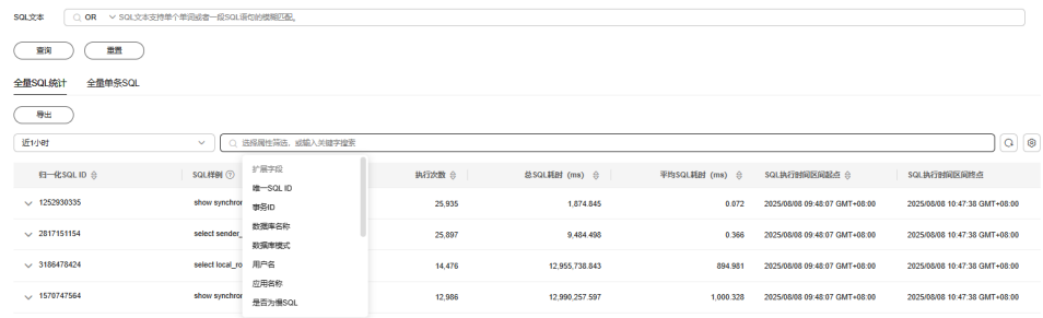
图 18-8 搜索条件
