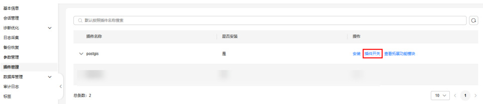
图 10-4 插件开关
