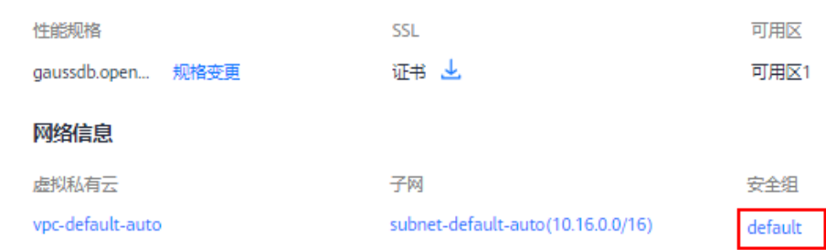
图 7-3 网络信息
