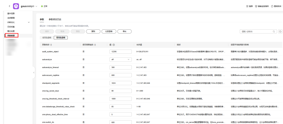
图 14-1 参数管理
