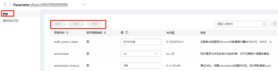
图 14-2 修改参数
