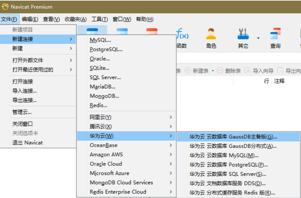
图 4-10 新建连接
