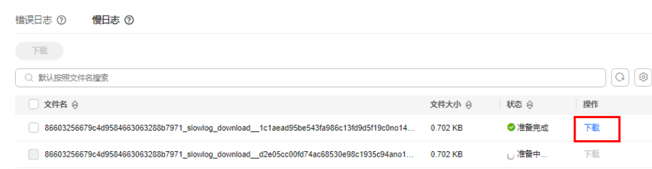
图 16-1 慢日志下载
