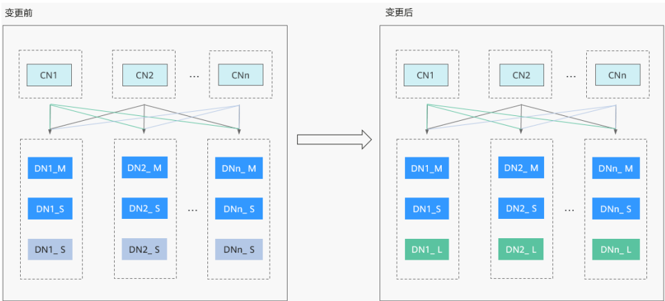
图 8-35 备 DN 节点变更为日志节点示意图
