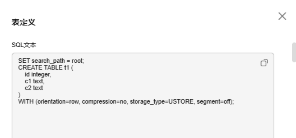
图 18-28 表定义
