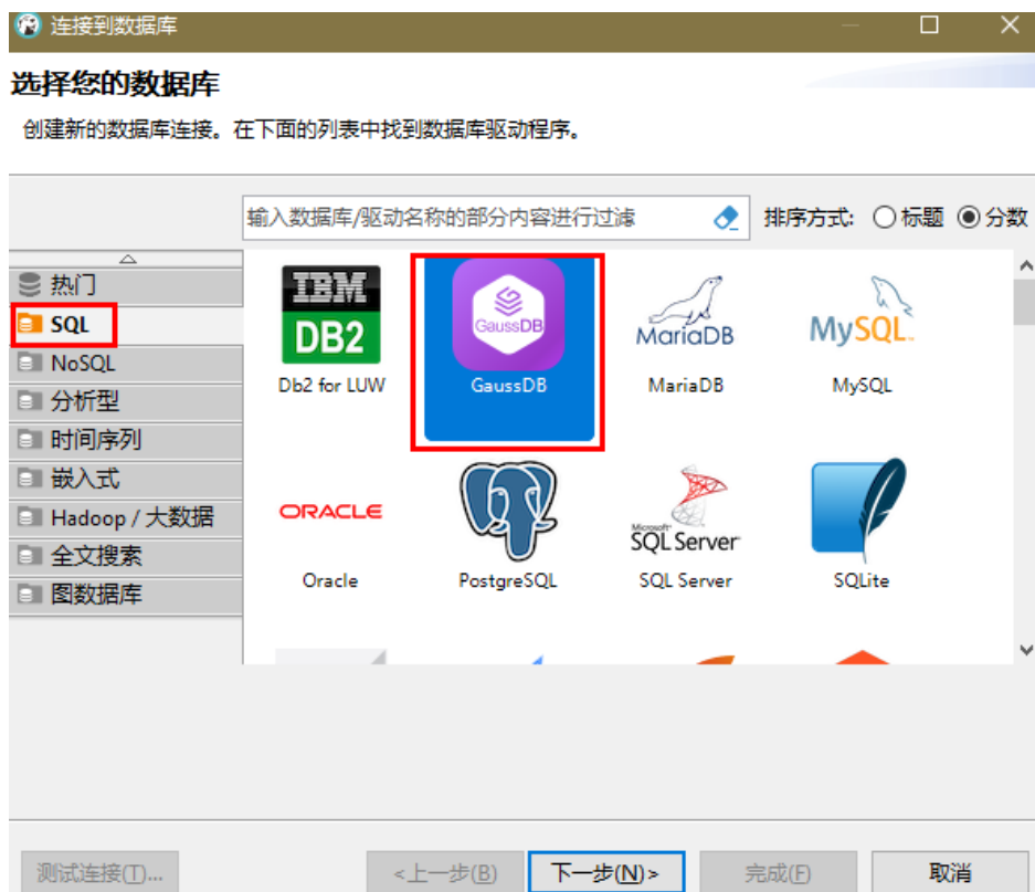
图 4-13 选择数据库
