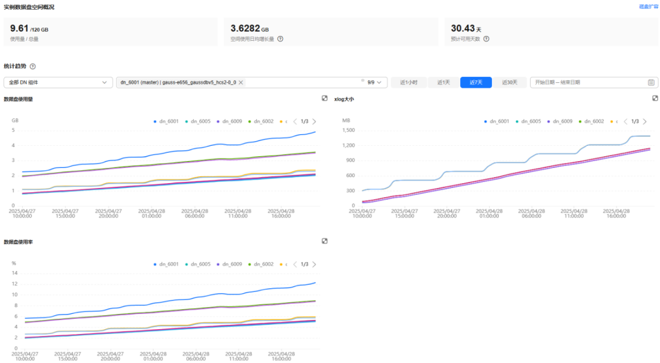
图 18-26 统计趋势
