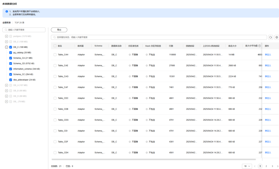
图 18-27 库表信息
