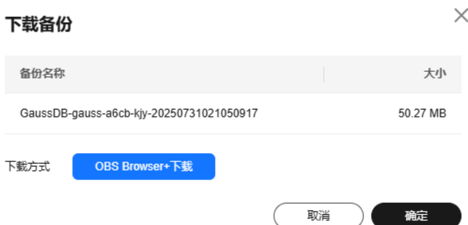
图 11-8 下载备份
