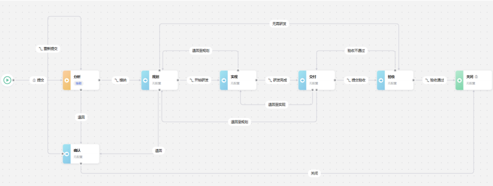
图 9-12 RR 状态流
