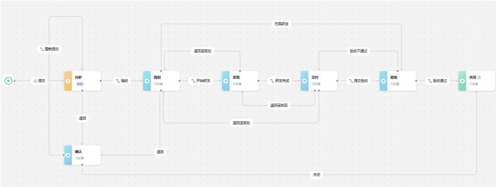
图 7-12 RR 状态流
