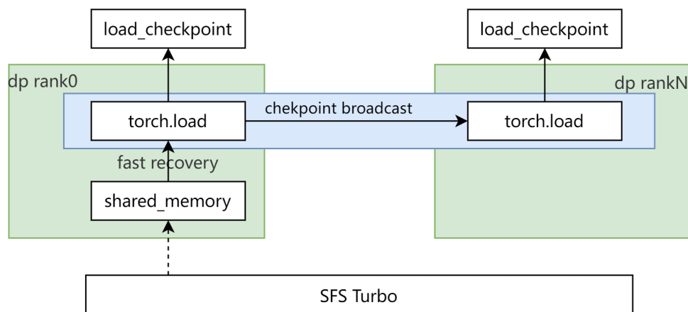
图 9-27 加载 checkpoint 流程
