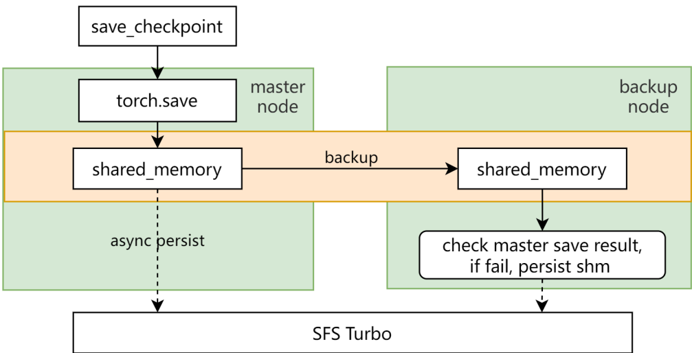
图 9-26 保存 checkpoint 流程
