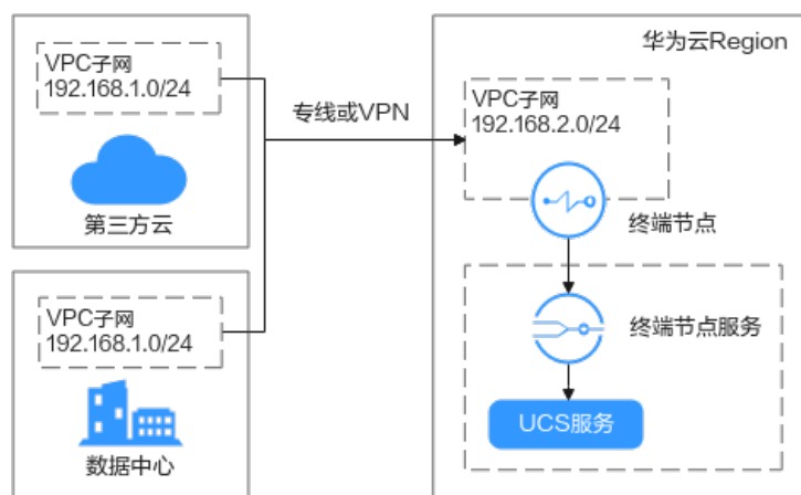
图 1-18 私网接入原理
