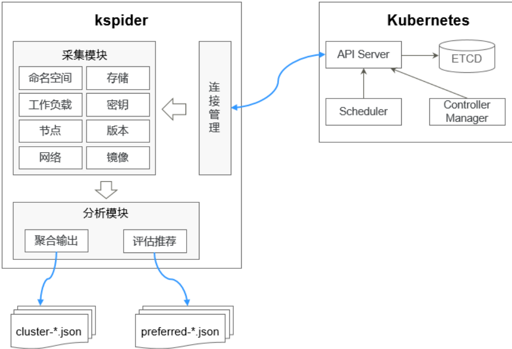
图 12-7 kspider 架构
