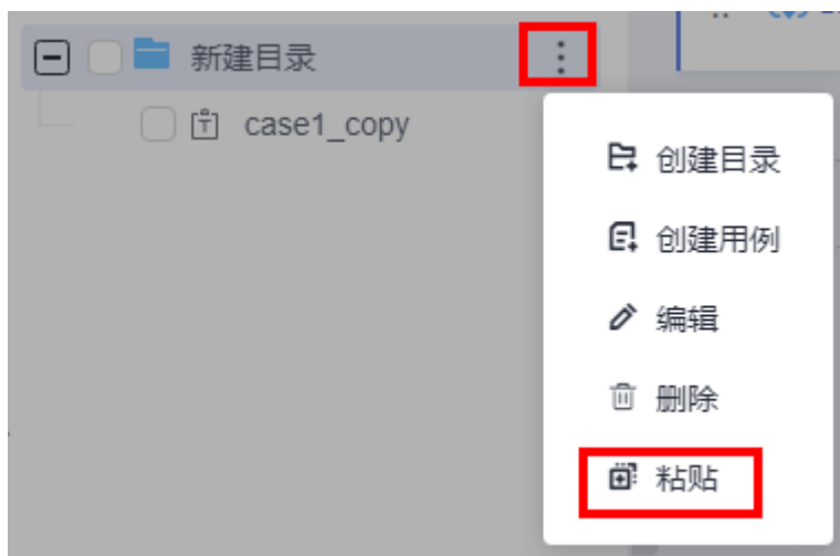
图 6-17 粘贴用例
