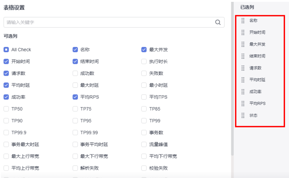
图 8-2 表格设置
