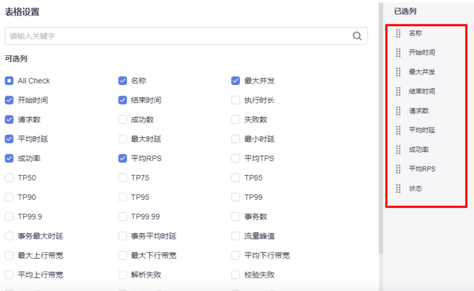
图 8-1 表格设置
