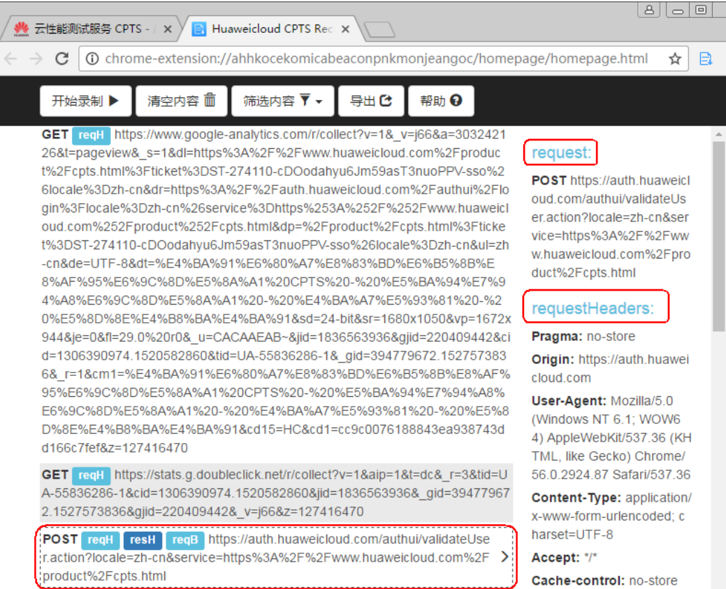
图 9-3 选择请求
