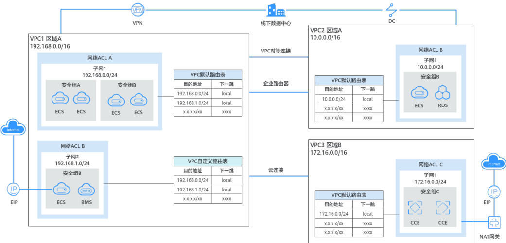
图 2-1 VPC 产品架构
