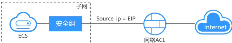
图 7-12 EIP 网络示意图
